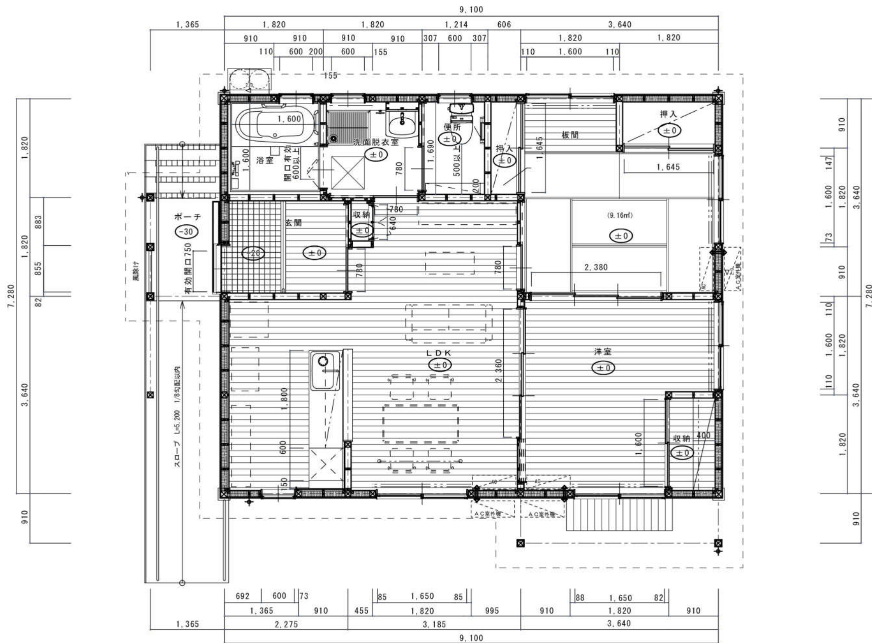
平屋建 2LDK 1階 平面図
