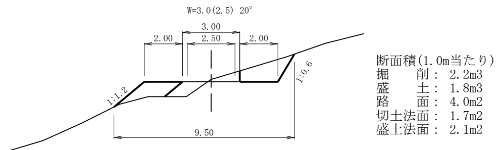
横断図 (D-2)
