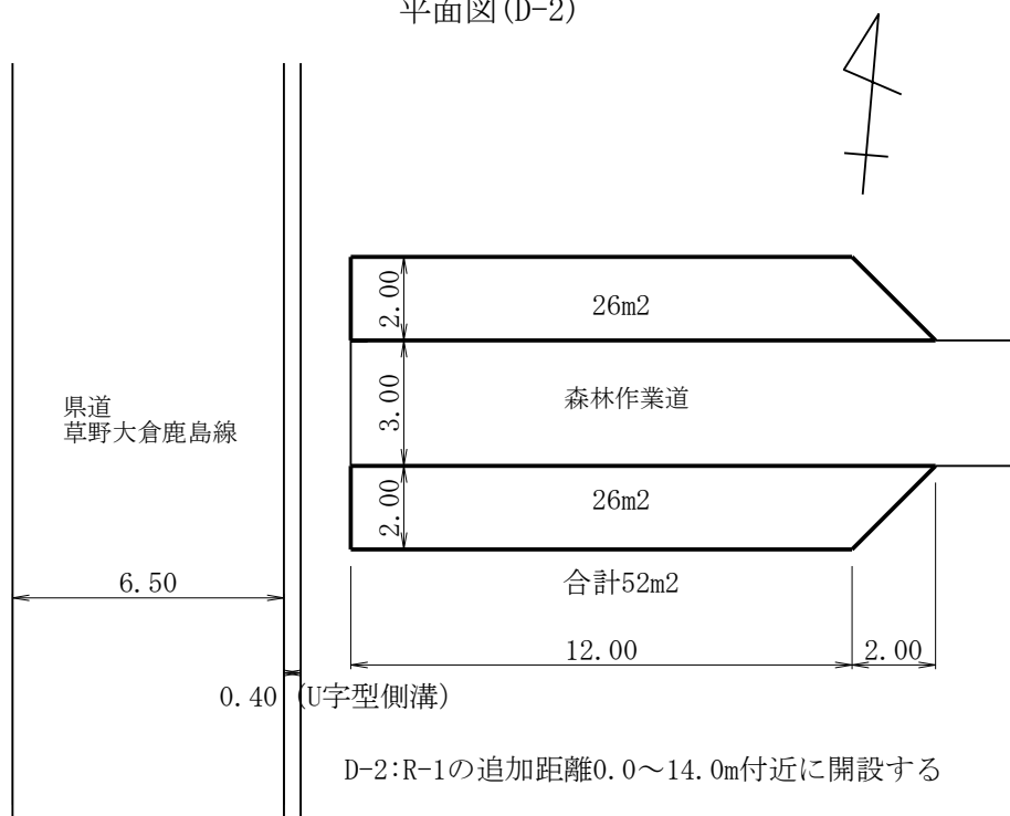
平面図 (D-2)
