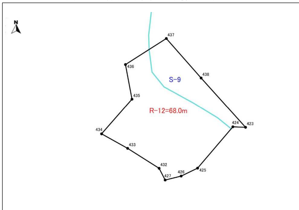
図表 1-12-1 平面図(地区番号 : S-9 面積 : 0.15ha)
