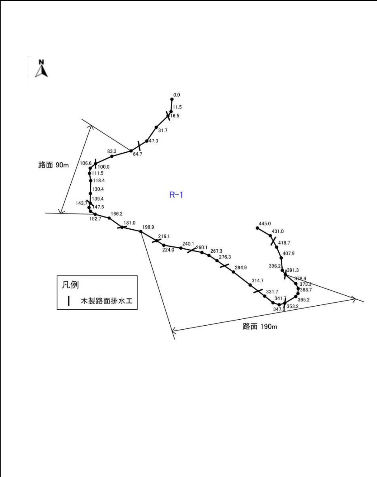
図表 4-1-1 R-1 の平面図(1)
