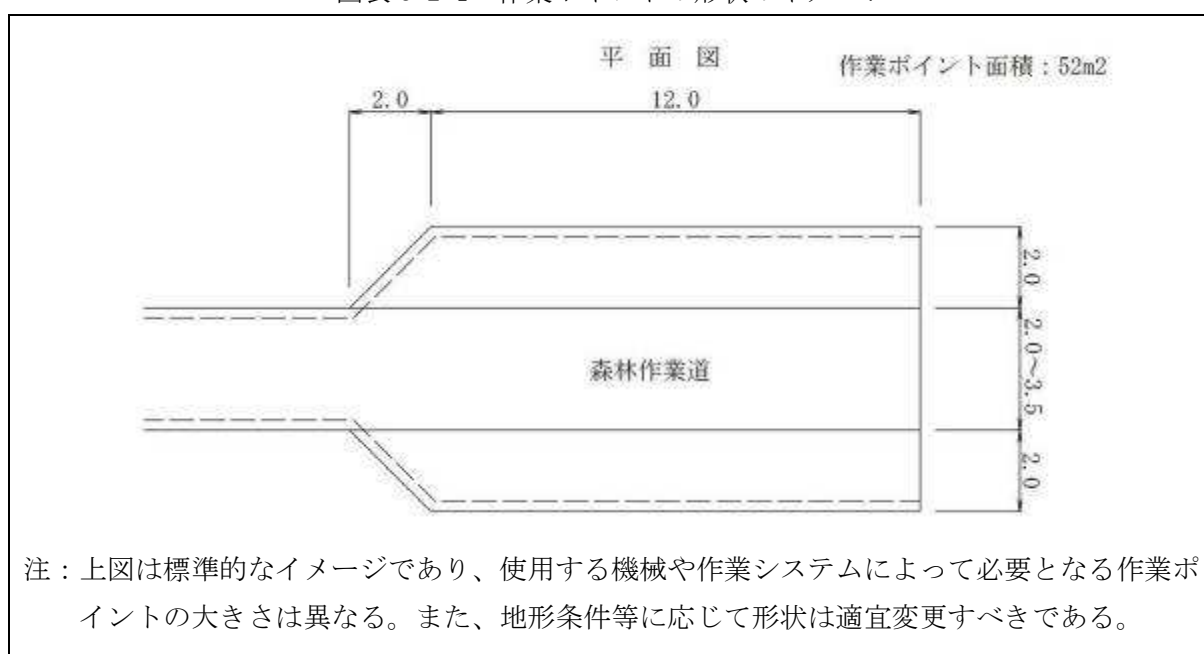
図表 5-2-1 作業ポイントの形状のイメージ
