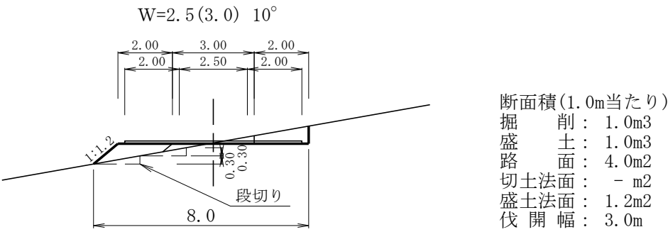
作業ポイント横断図(D-6)
