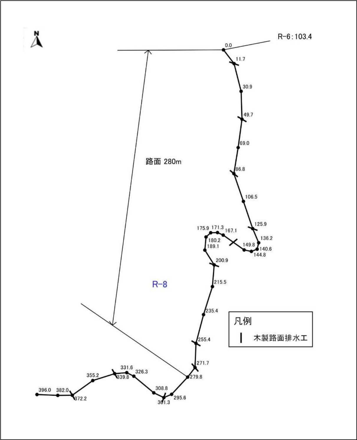
図表 4-8-1 R-8 の平面図(1)
