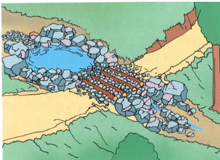
図表 5-1-12 洗い越しの例
