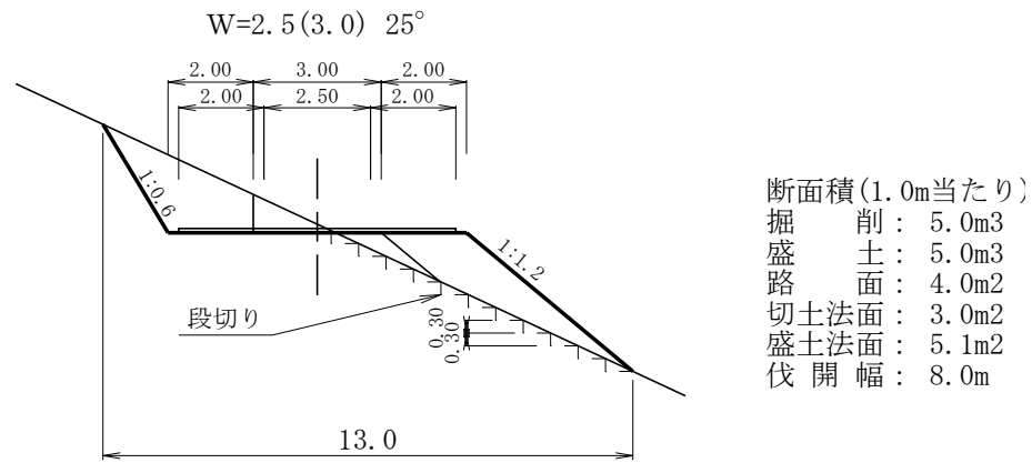
作業ポイント横断図(D-8)
