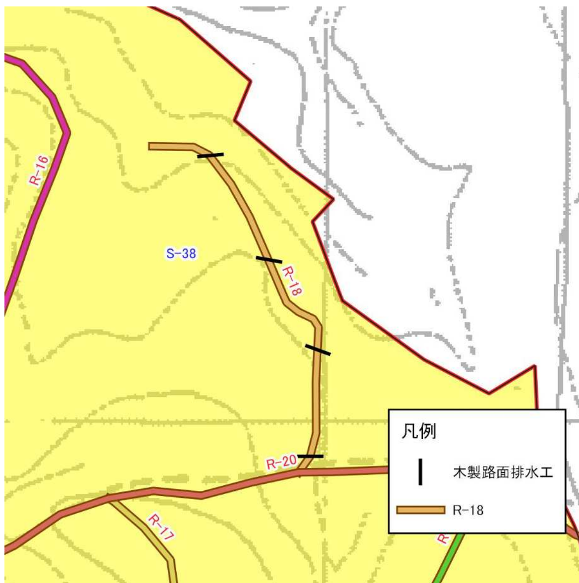
図表 4-18-3 R-18 の平面図(2)
