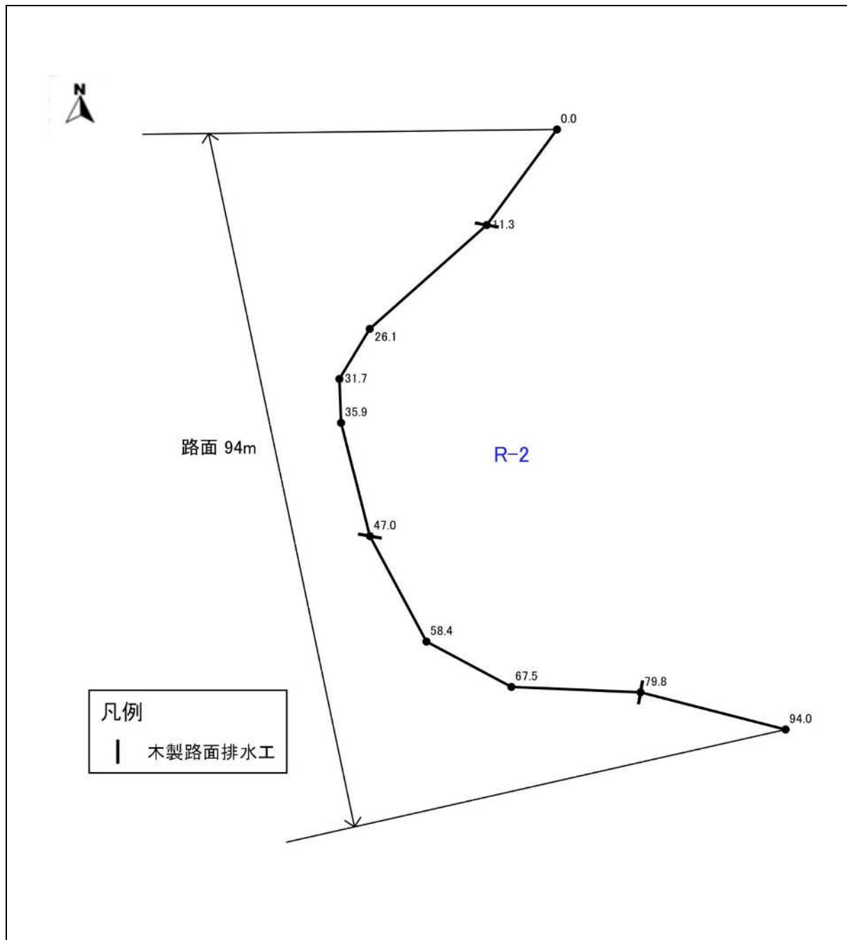
図表 4-2-1 R-2 の平面図(1)
