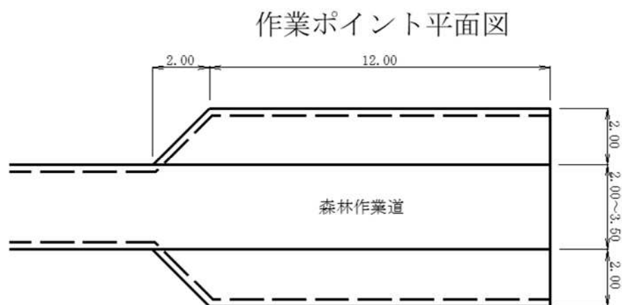
図表 5-13-2 D-10 標準平面図
