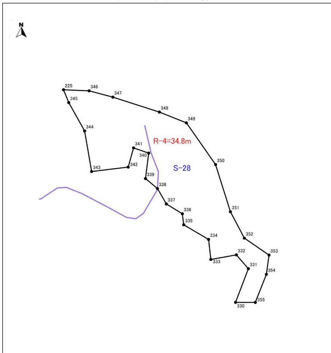
図表 1-31-1 平面図(地区番号：S-28 面積：0.34ha)
