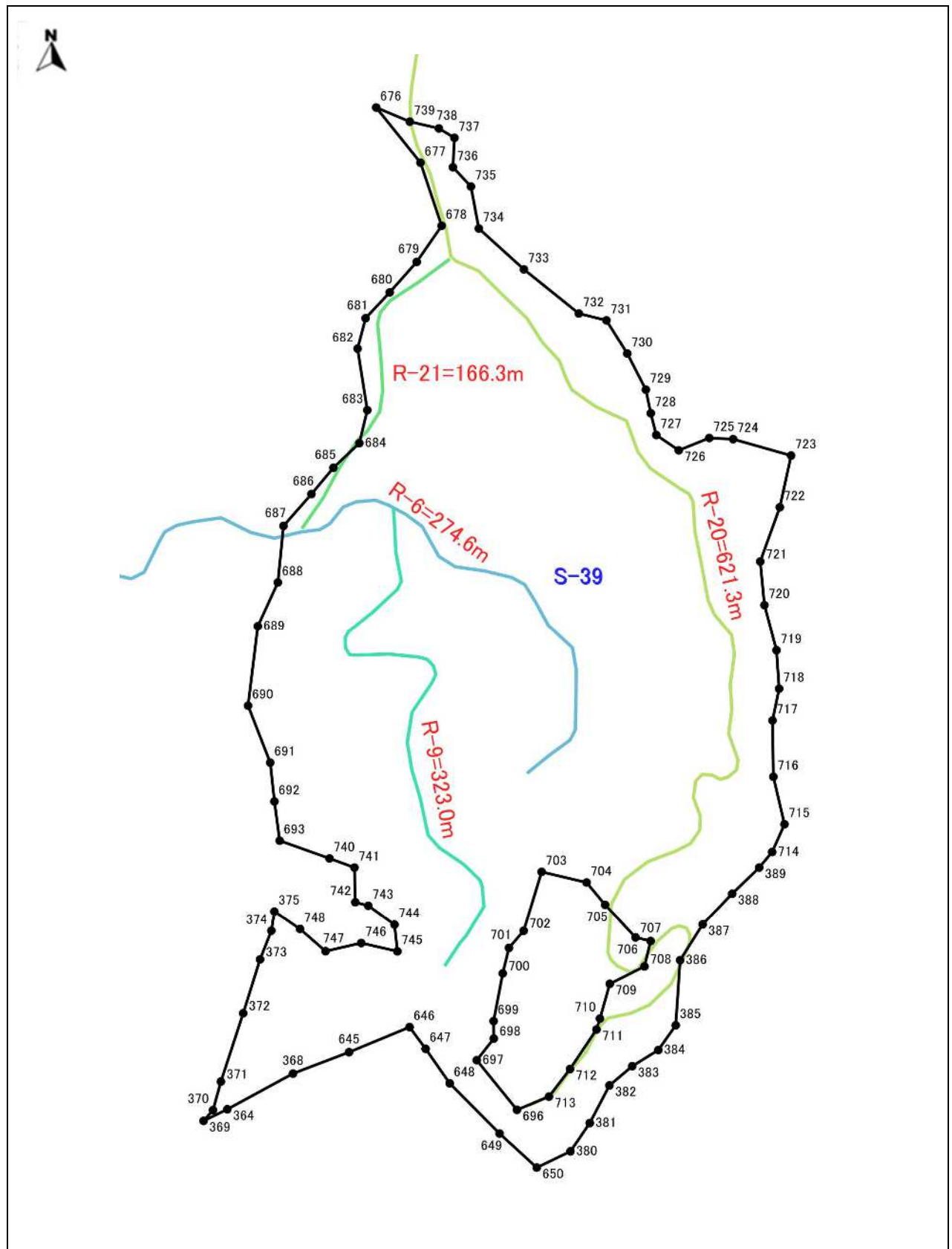
図表 1-42-1 平面図(地区番号：S-39 面積：9.38ha)
