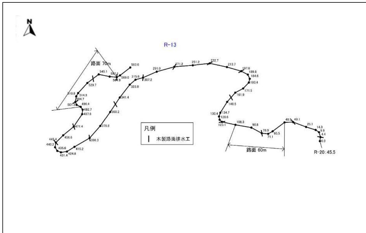
図表 4-13-1 R-13 の平面図(1)
