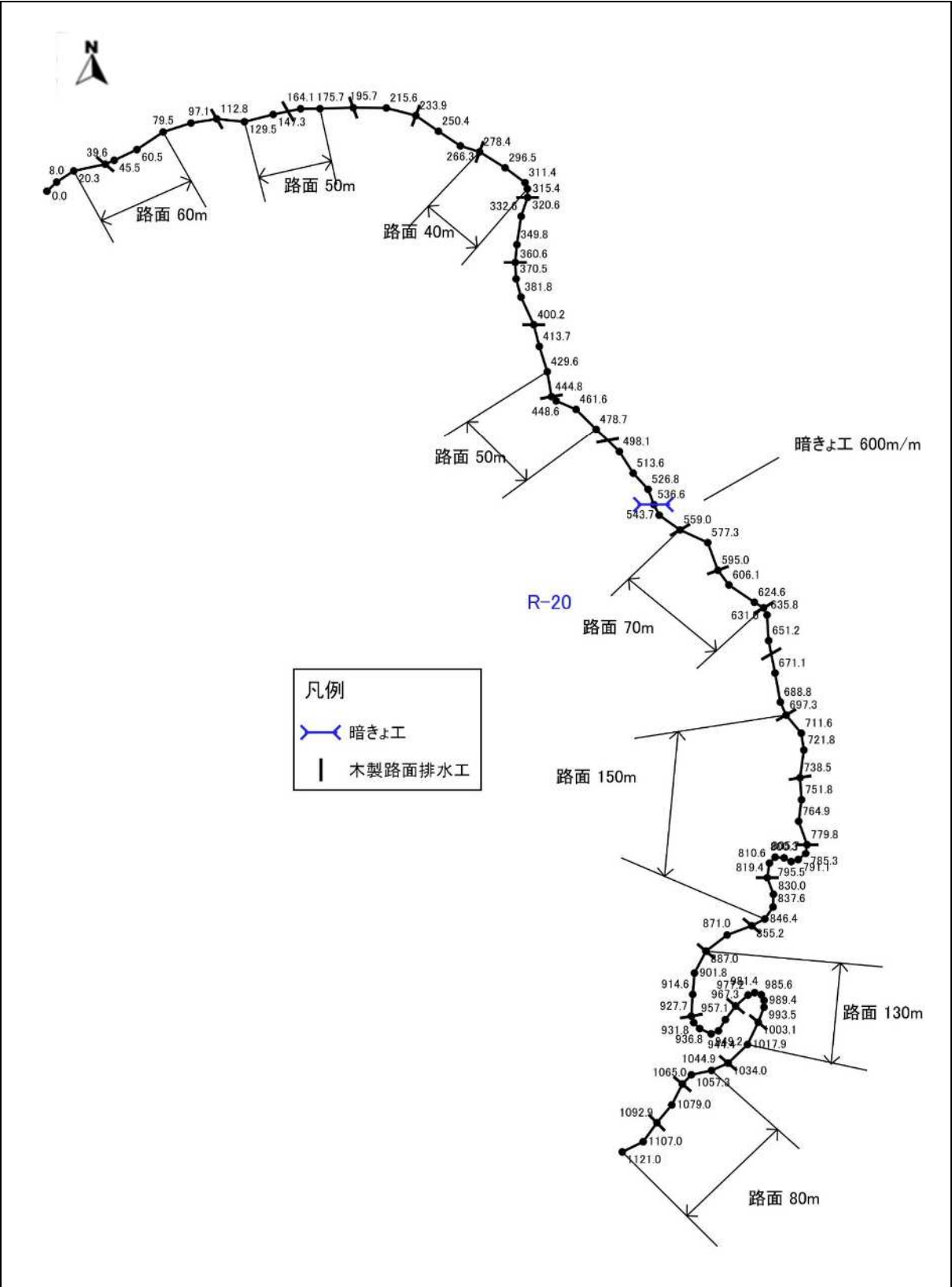
図表 4-20-1 R-20 の平面図(1)
