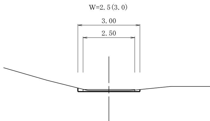
R-1標準横断図
