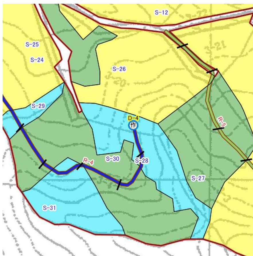
図表 5-7-1 D-4 平面図
