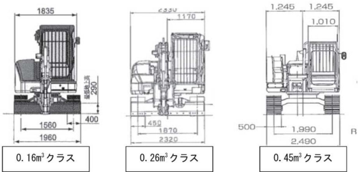
図表 5-1-4 ベースマシンの車幅の例
