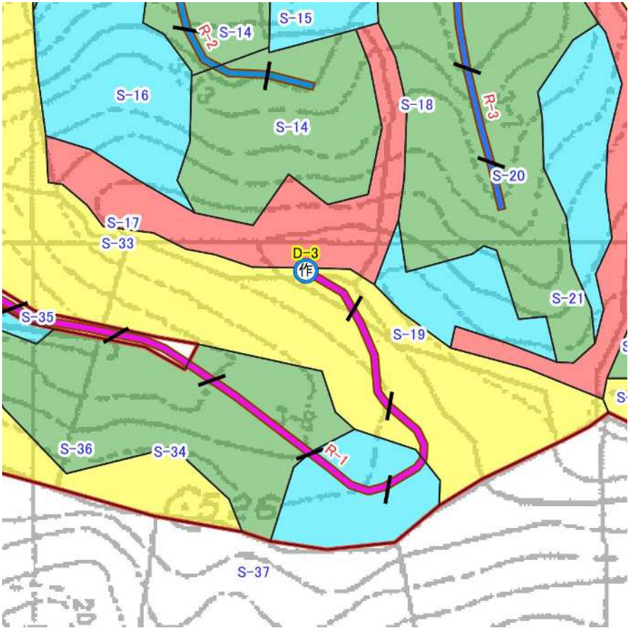
図表 5-6-1 D-3 平面図
