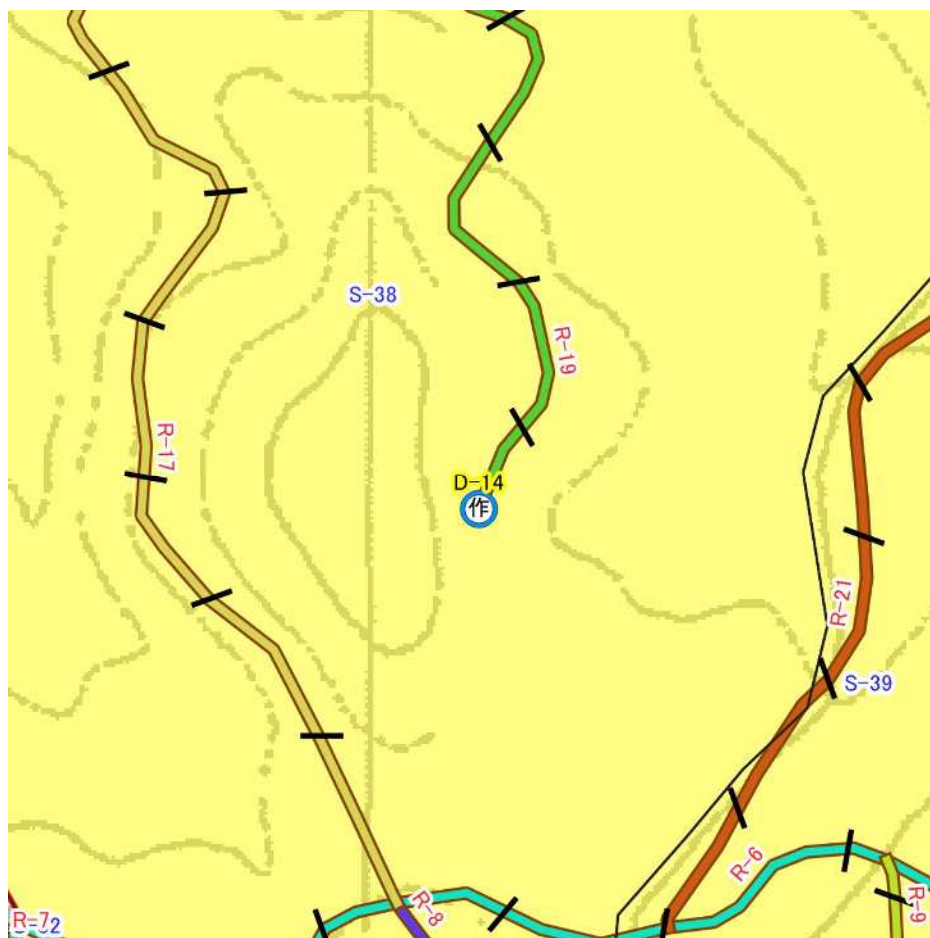
図表 5-17-1 D-14 平面図
