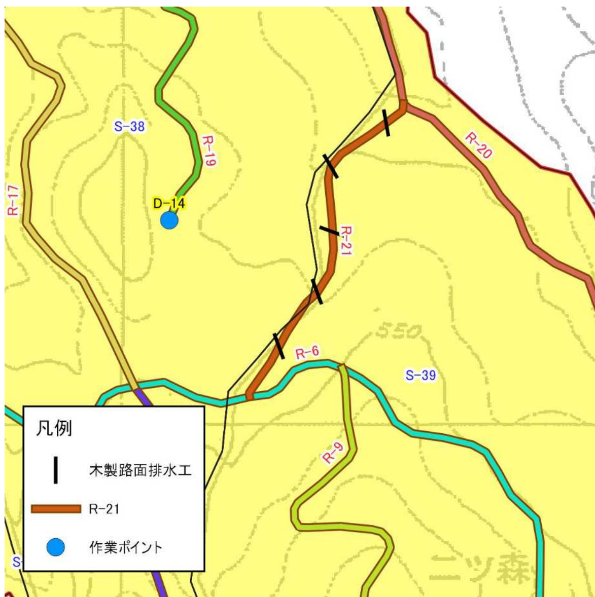
図表 4-21-3 R-21 の平面図(2)
