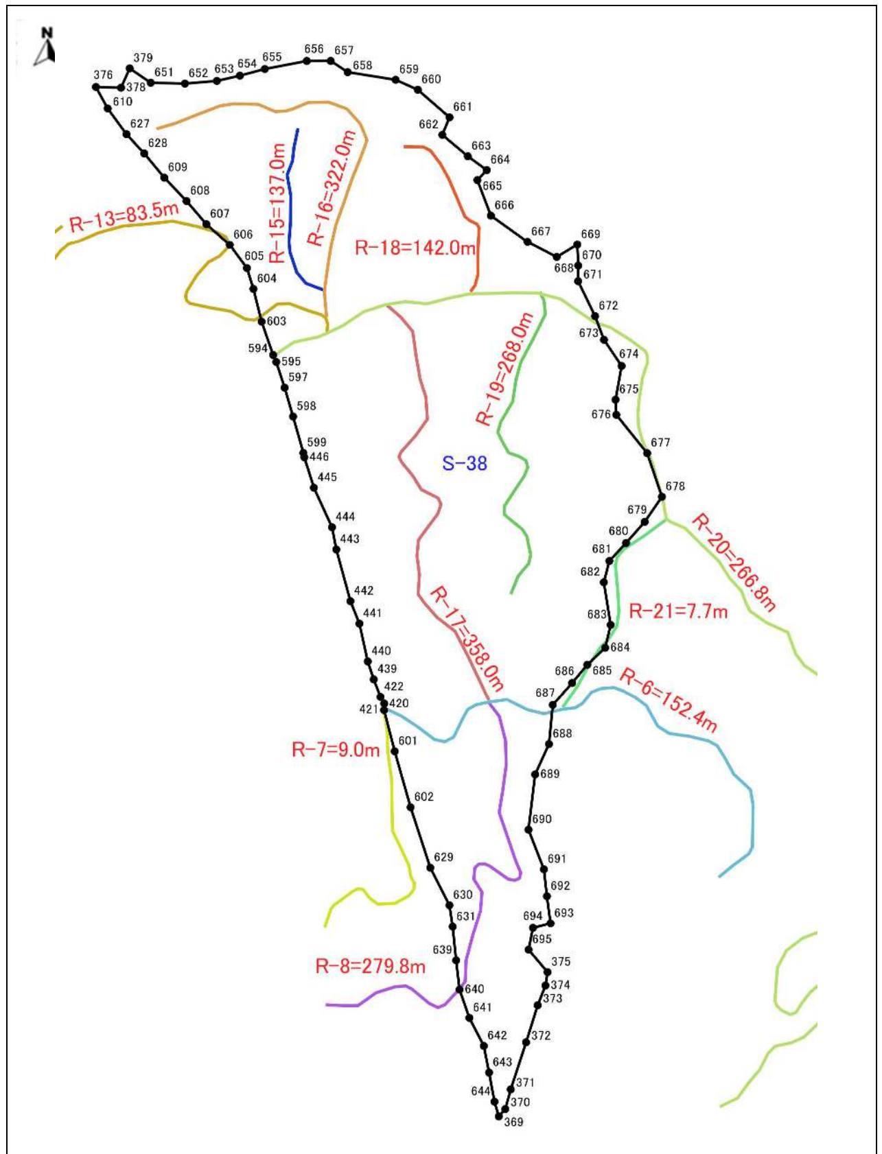
図表 1-41-1 平面図(地区番号：S-38 面積：13.64ha)
