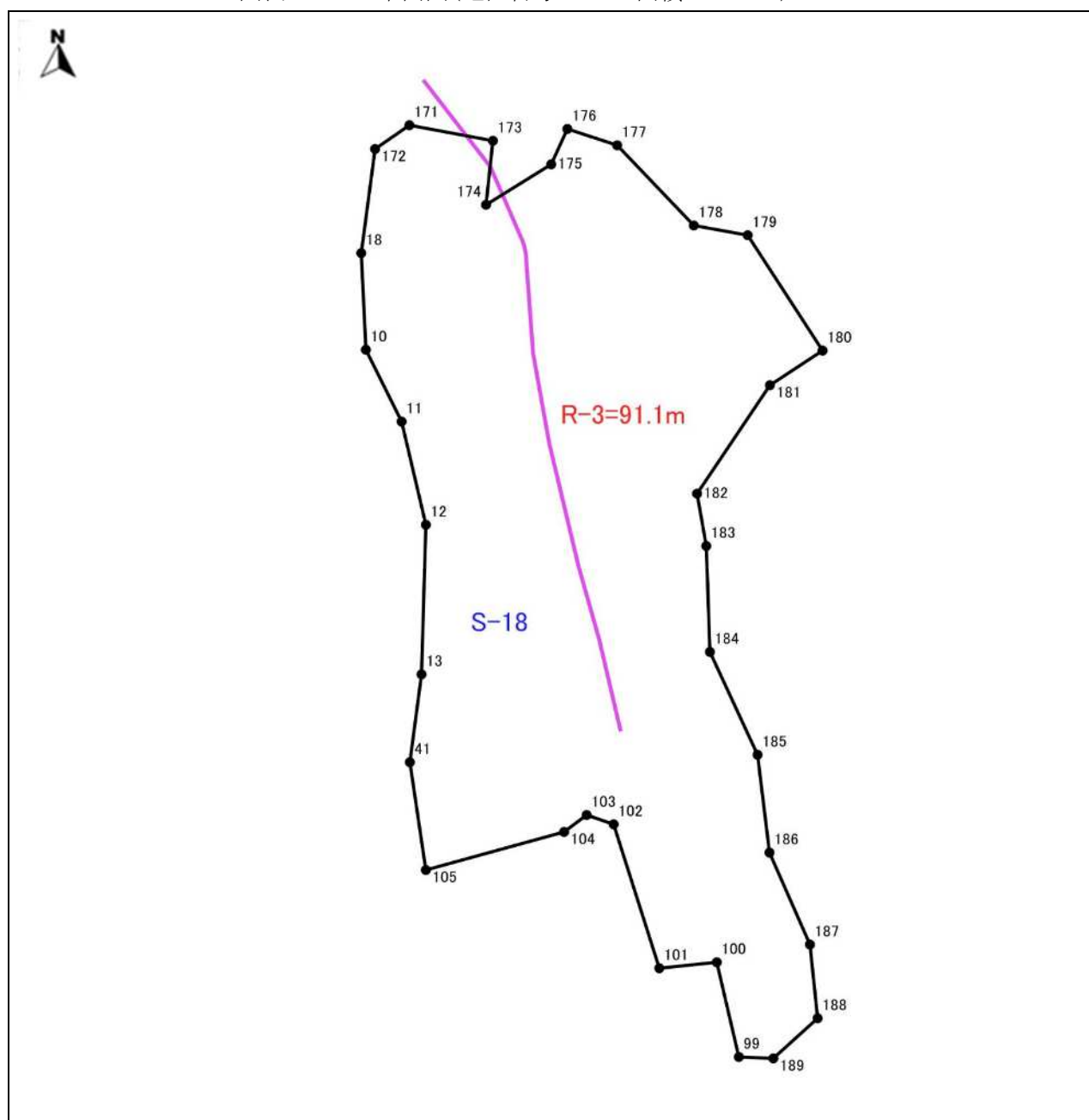
図表 1-21-1 平面図(地区番号：S-18 面積：0.61ha)
