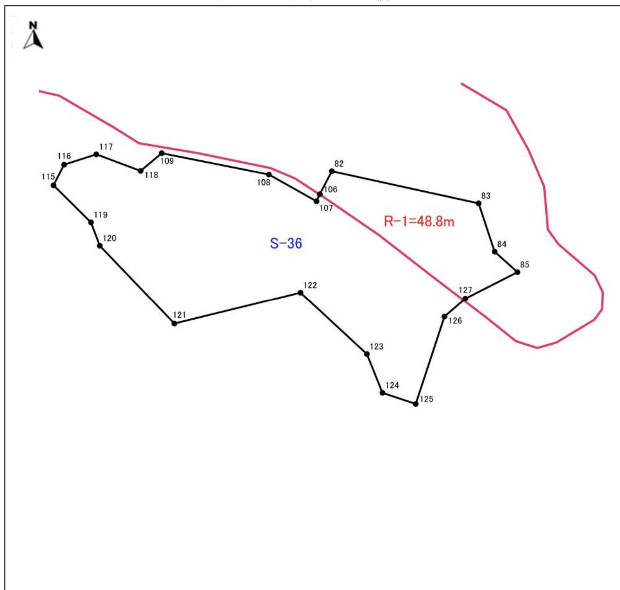
図表 1-38-1 平面図(地区番号：S-36 面積：0.42ha)
