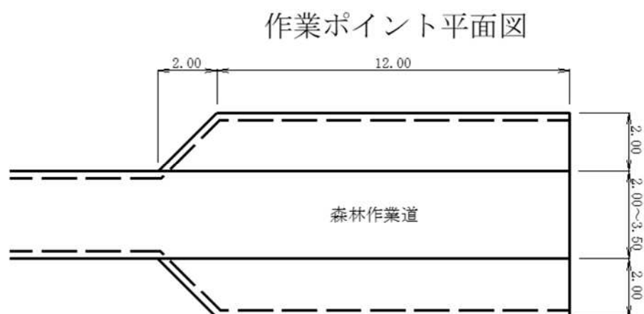
図表 5-17-2 D-14 標準平面図
