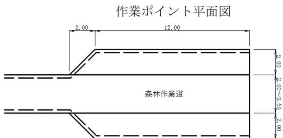
図表 5-18-2 D-15 標準平面図
