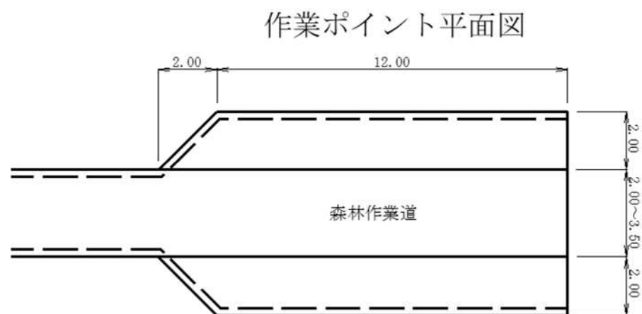
図表 5-10-2 D-7 標準平面図
