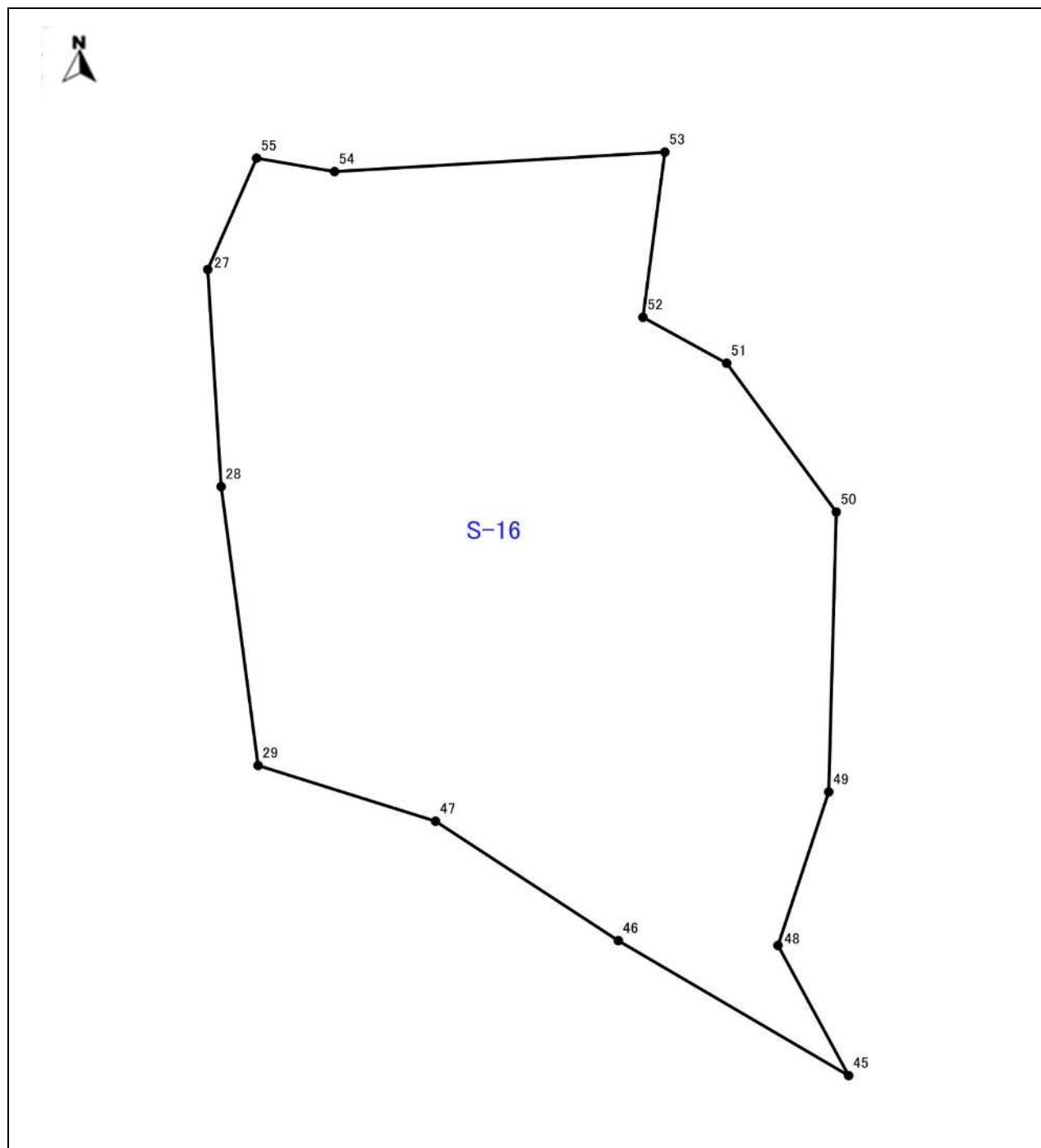
図表 1-19-1 平面図(地区番号 : S-16 面積 : 0.25ha)
