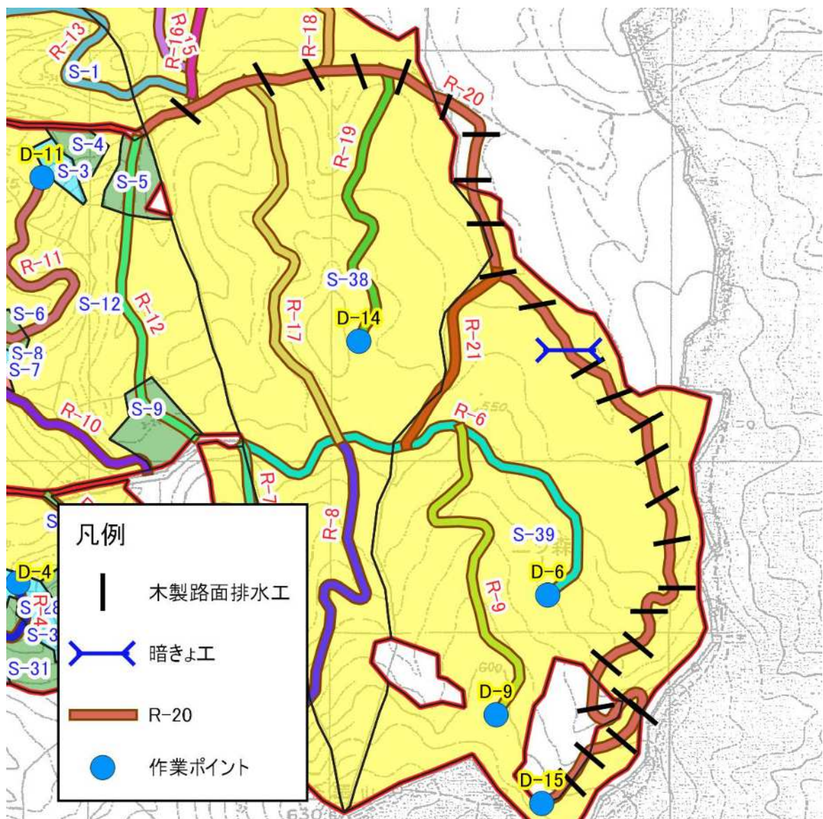
図表 4-20-3 R-20 の平面図(2)
