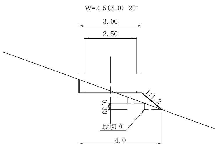
R-1標準横断図
