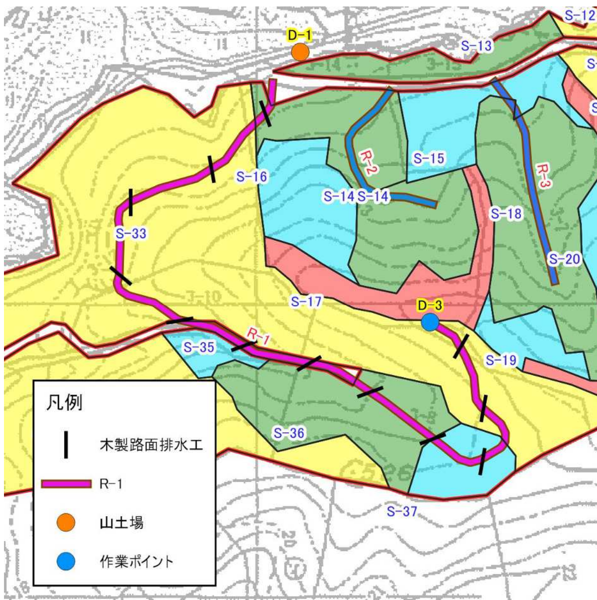
図表 4-1-3 R-1 の平面図(2)
