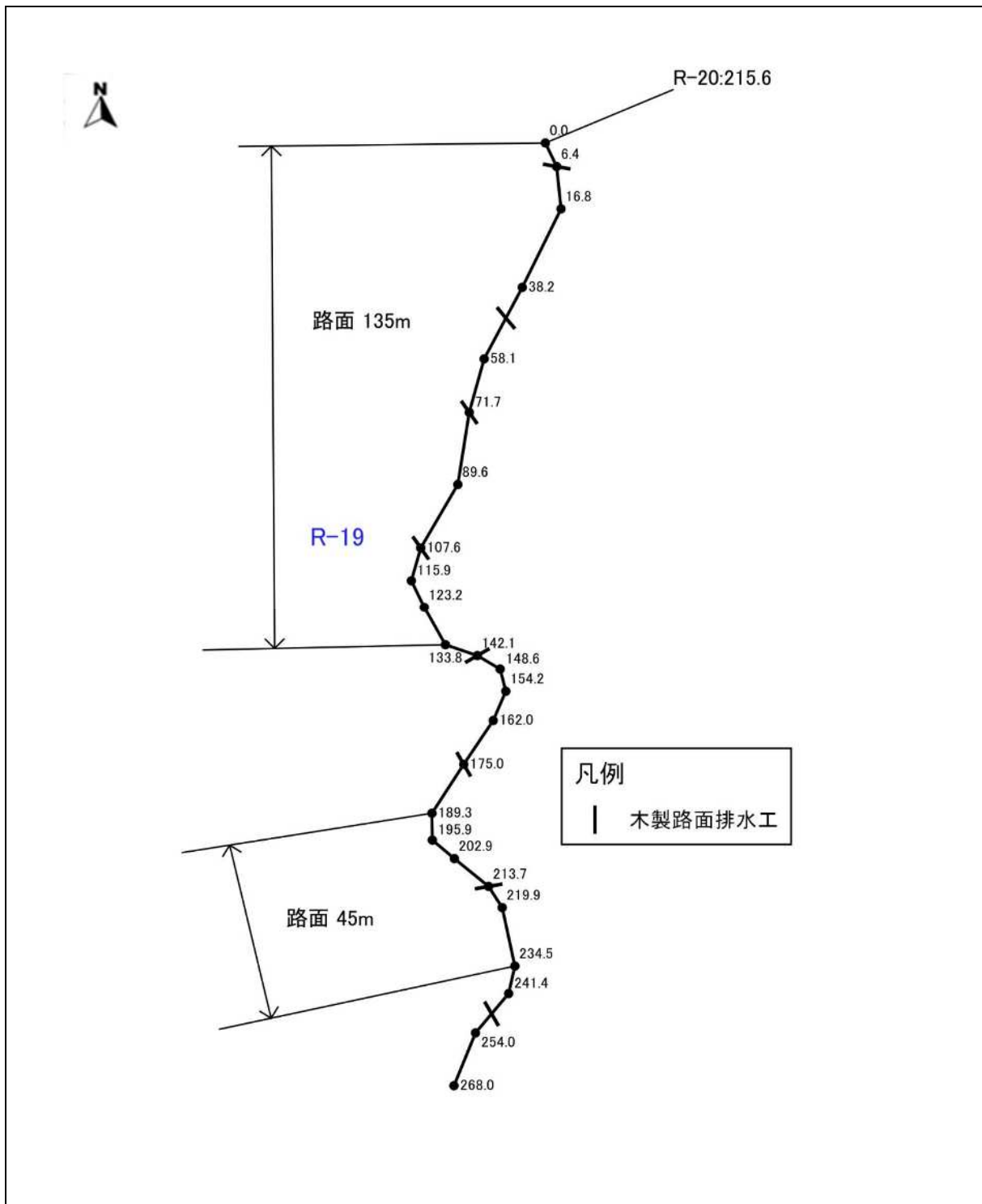
図表 4-19-1 R-19 の平面図(1)
