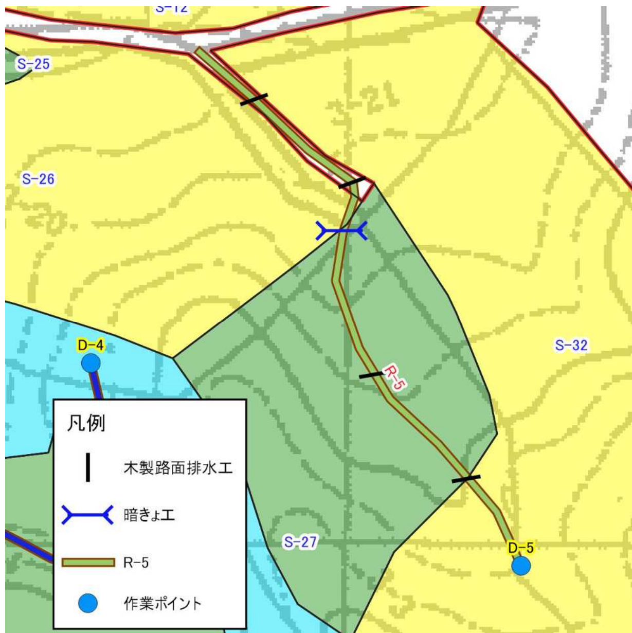
図表 4-5-3 R-5 の平面図(2)
