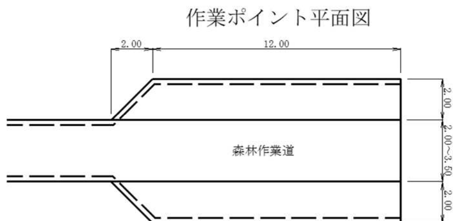
図表 5-16-2 D-13 標準平面図
