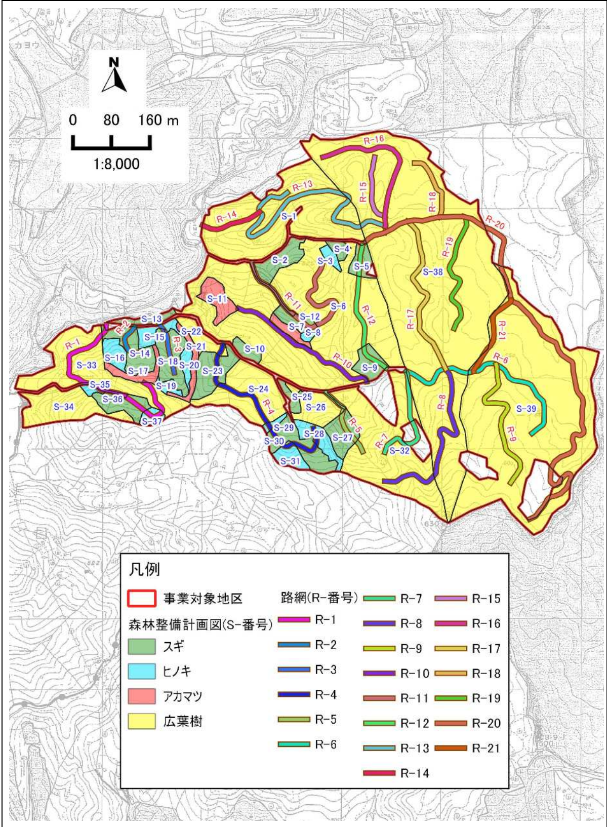
図表 5-4-1 路網配置計画図
