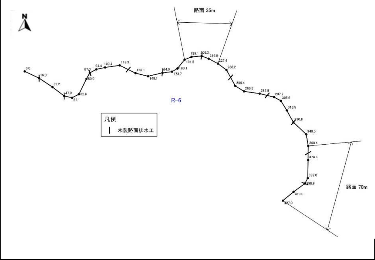
図表 4-6-1 R-6 の平面図 (1)
