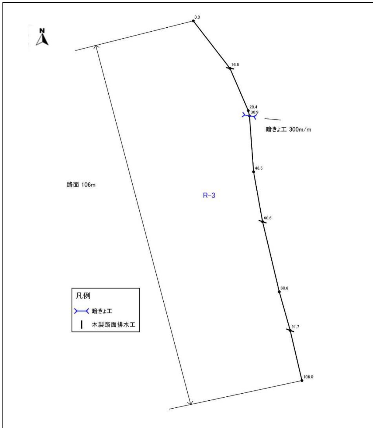
図表 4-3-1 R-3 の平面図(1)
