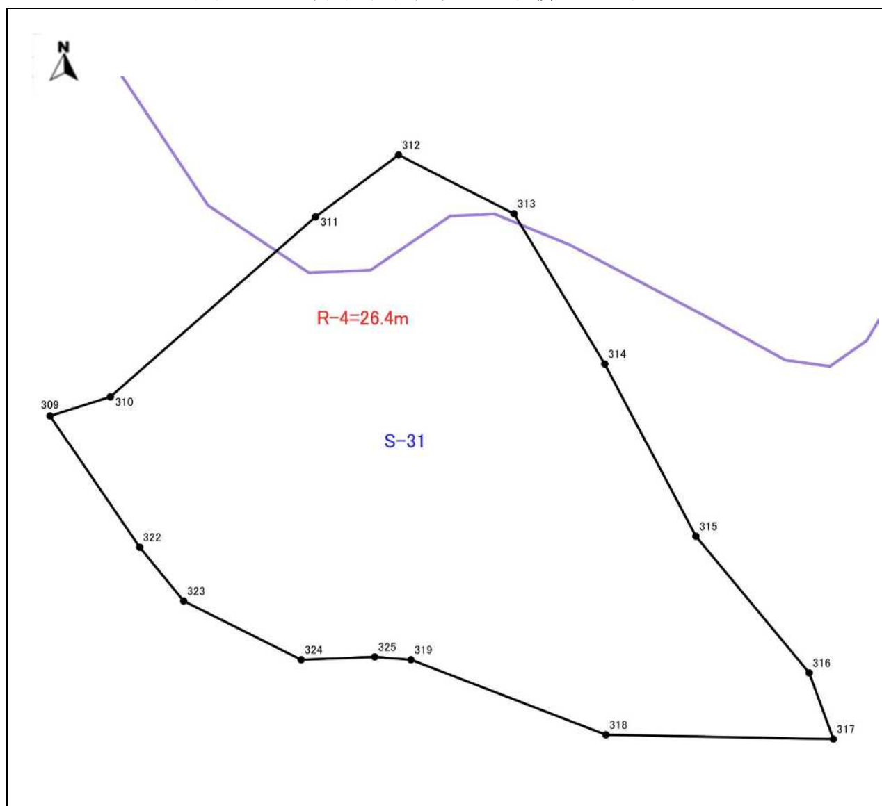
図表 1-34-1 平面図(地区番号：S-31 面積：0.26ha)
