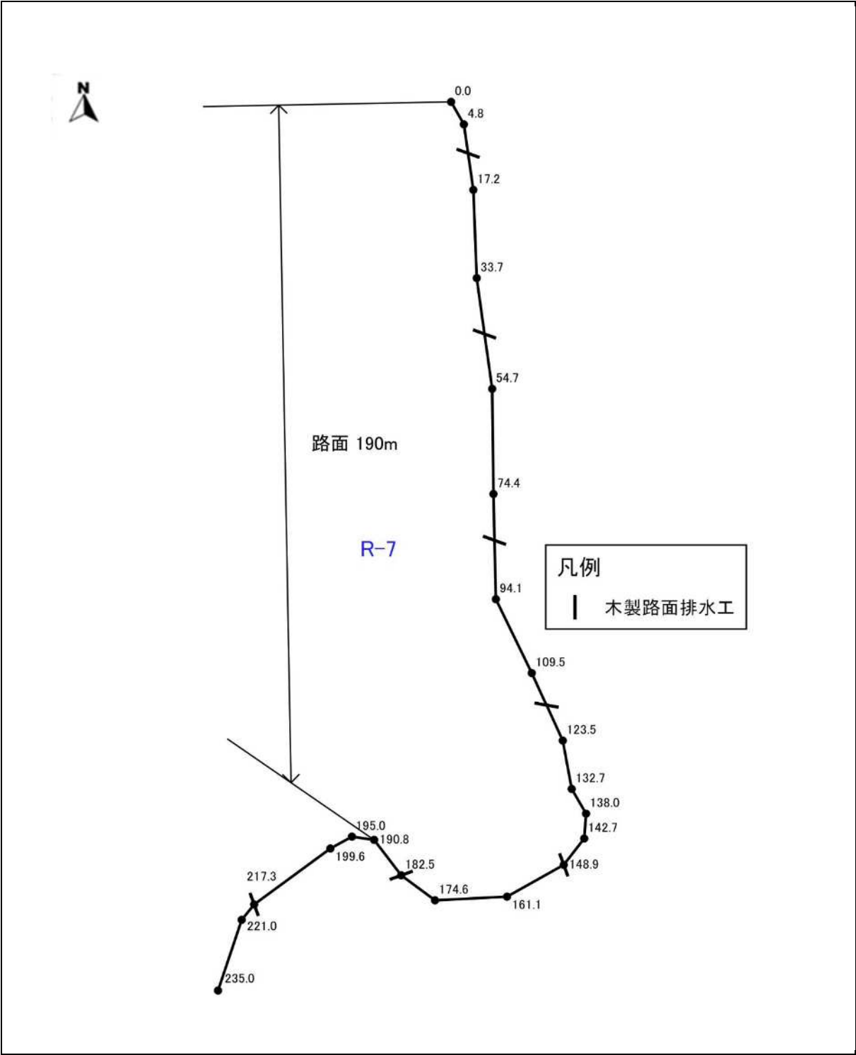
図表 4-7-1 R-7 の平面図(1)
