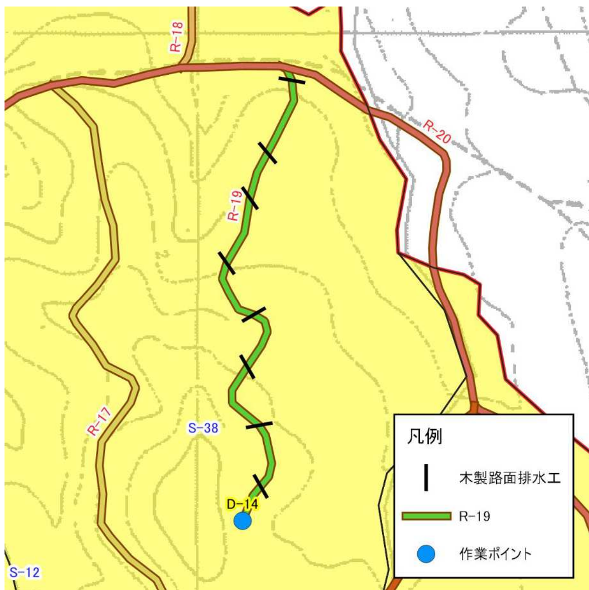
図表 4-19-3 R-19 の平面図(2)
