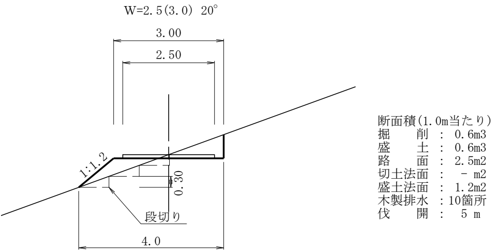
R-17標準横断面図
