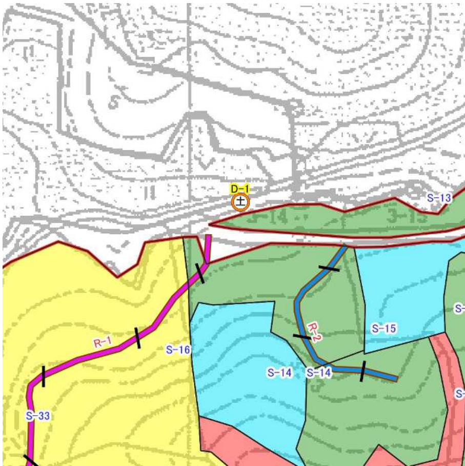
図表 5-4-1 D-1 平面図
