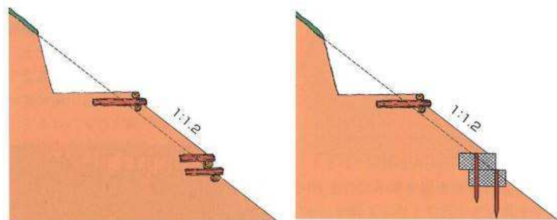
丸太組工
