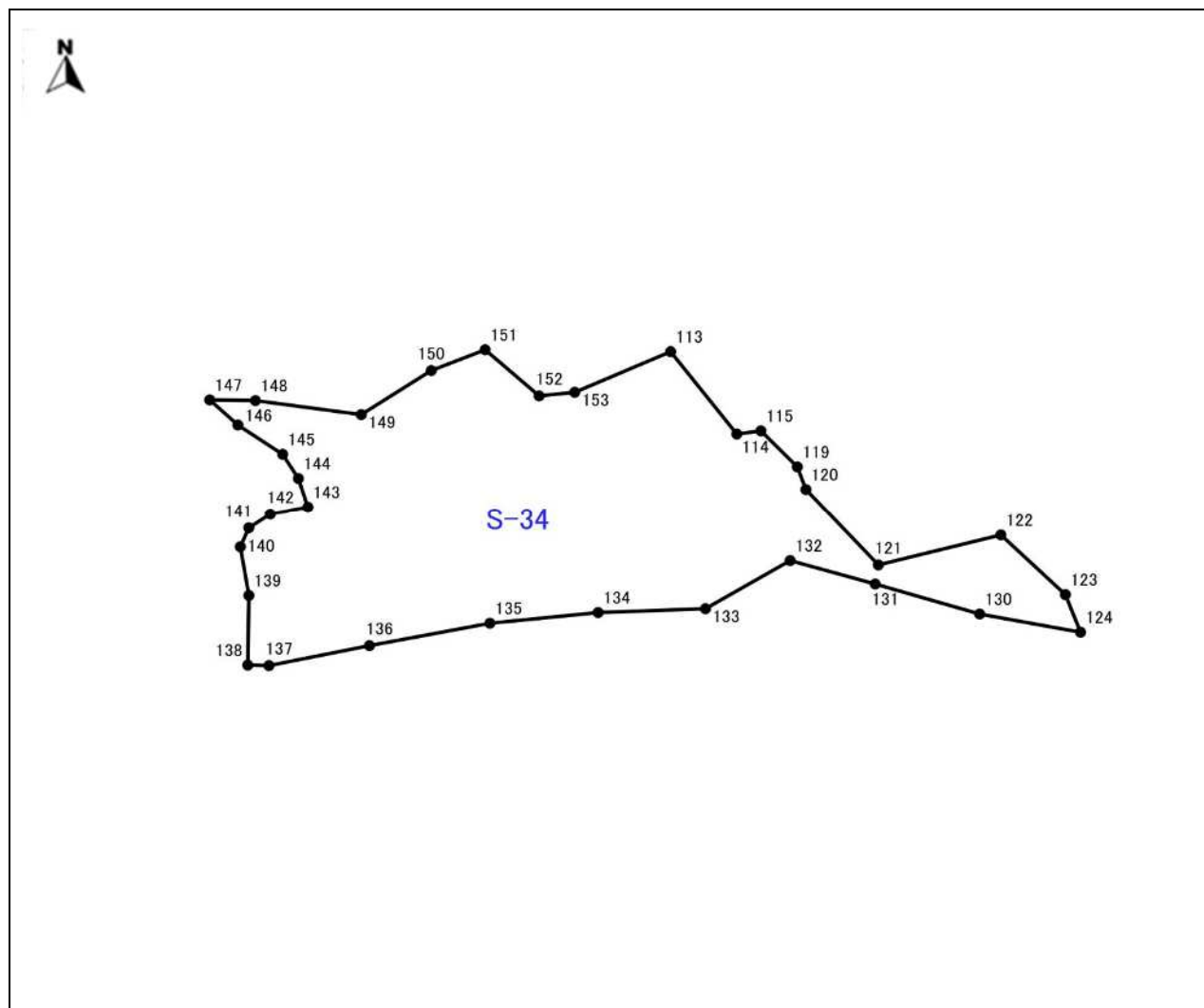
図表 1-37-1 平面図(地区番号：S-34 面積：1.08ha)
