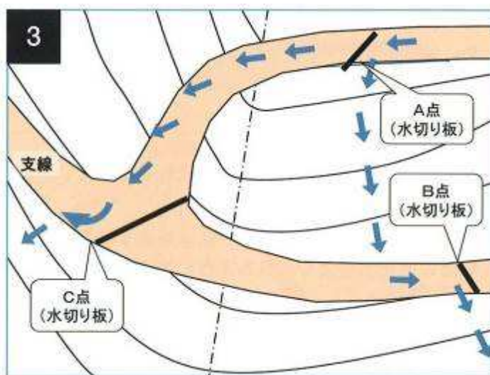
図表 5-1-8 曲線部の手前での排水の例
