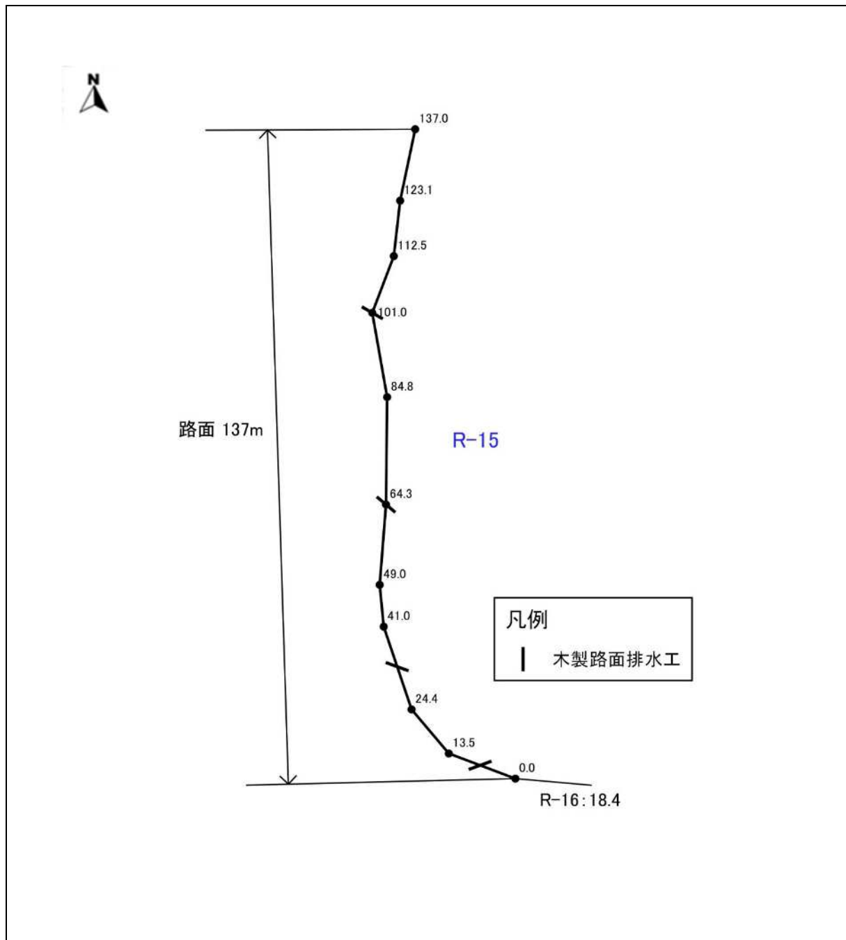
図表 4-15-1 R-15 の平面図(1)
