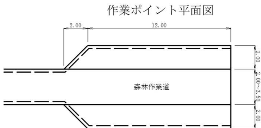
図表 5-9-2 D-6 標準平面図
