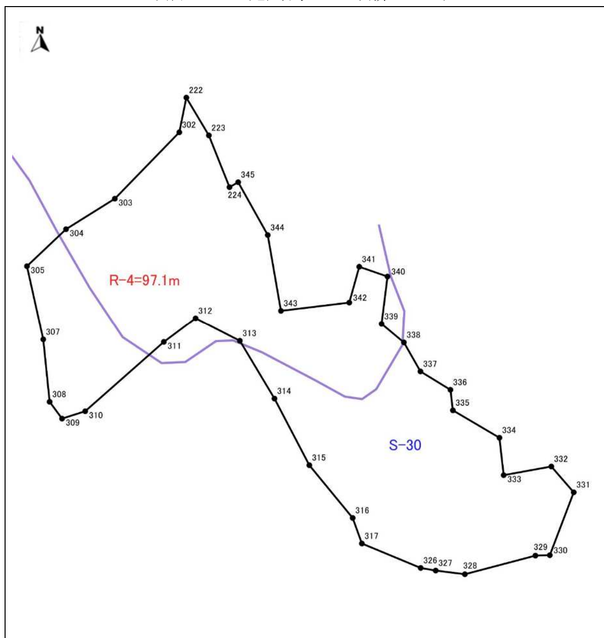
図表 1-33-1 (地区番号 : S-30 面積 : 0.66ha)
