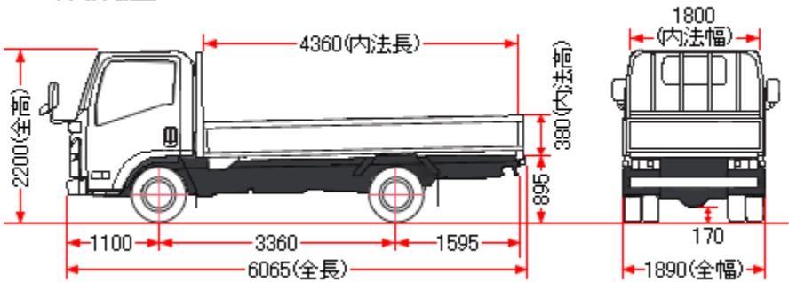
図表 5-1-5 4t 積みトラックの仕様例
