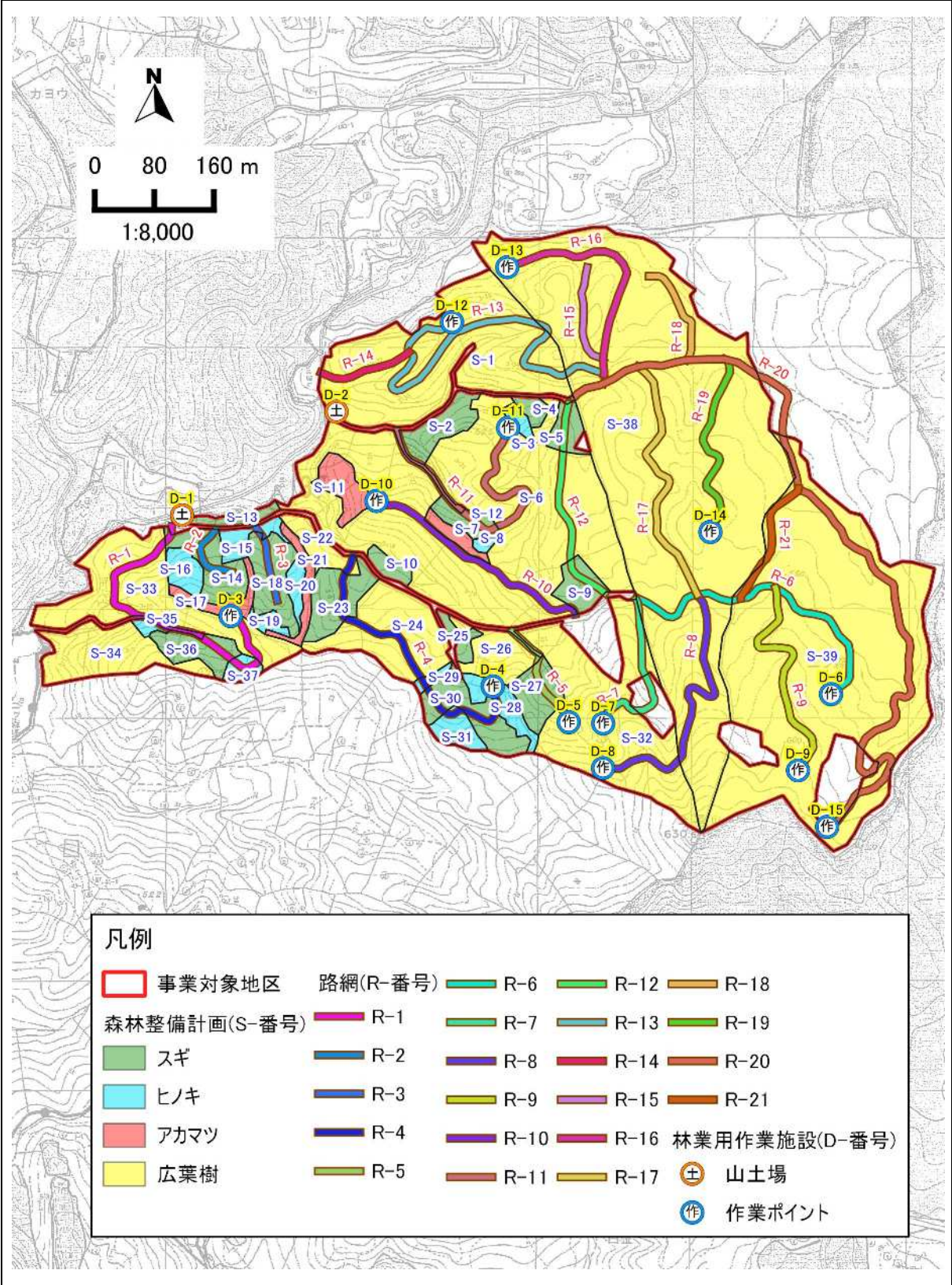
図表 6-1 林業用作業施設計画図
