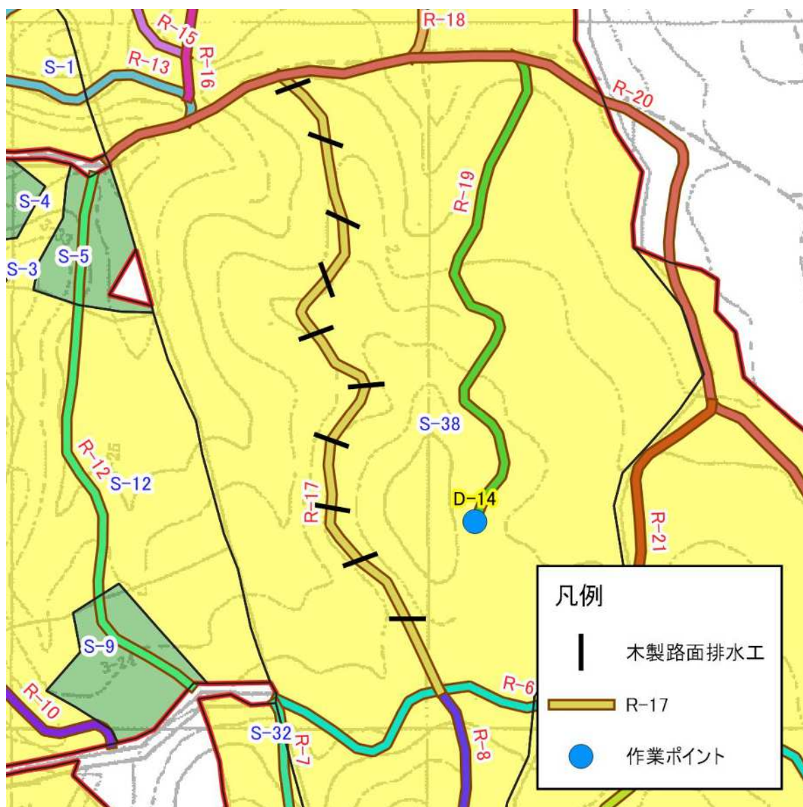
図表 4-17-3 R-17 の平面図(2)
