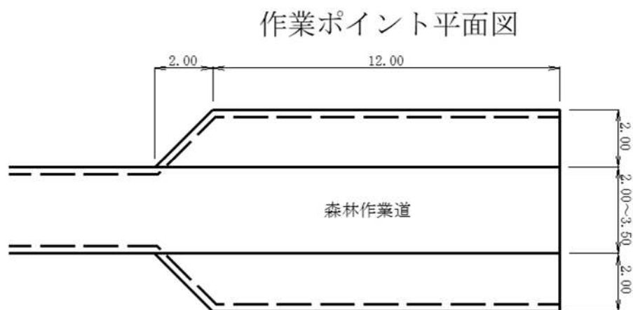
図表 5-12-2 D-9 標準平面図
