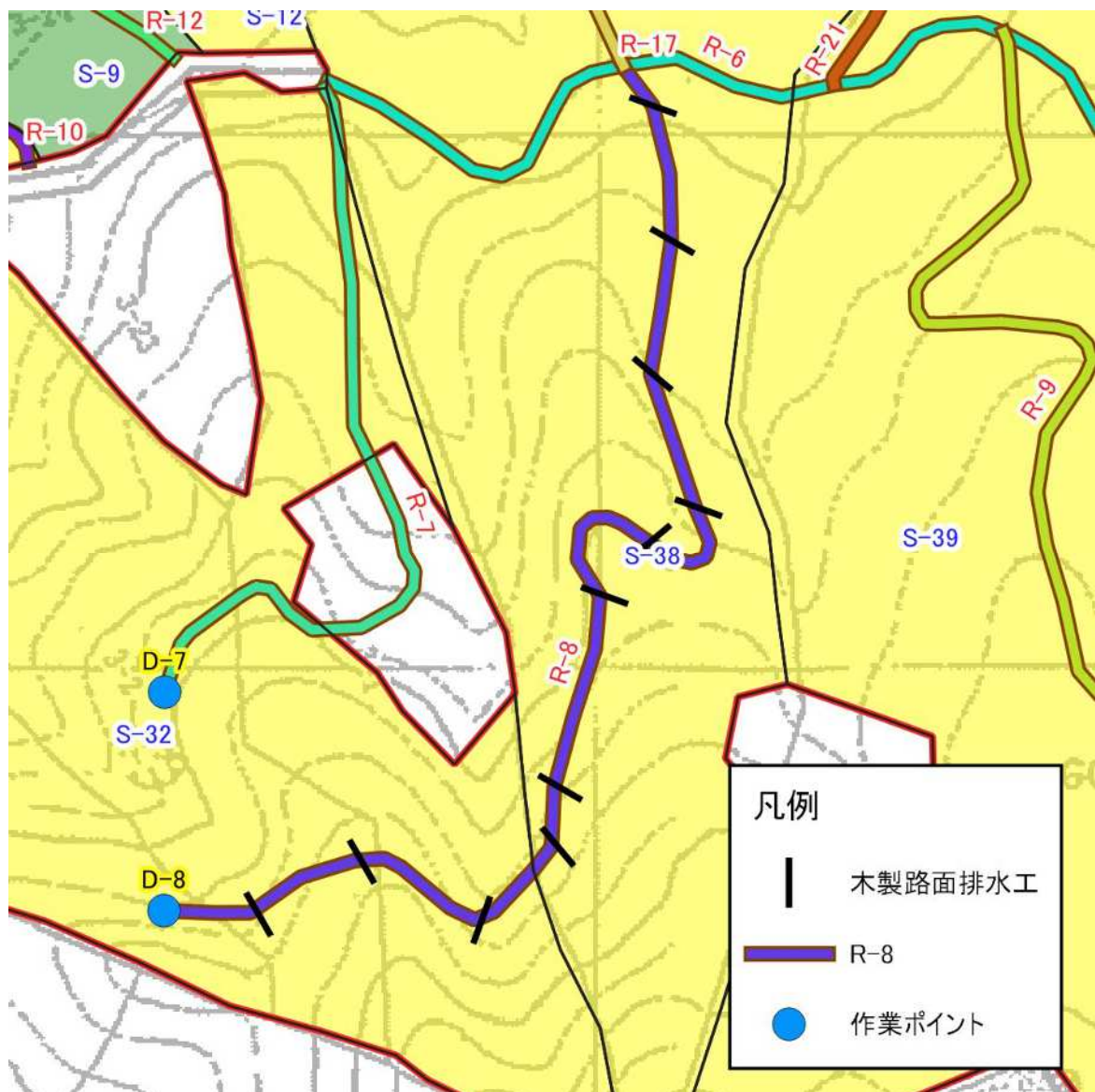
図表 4-8-3 R-8 の平面図(2)
