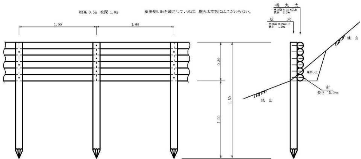
図表 3-2-1 丸太柵工標準図
