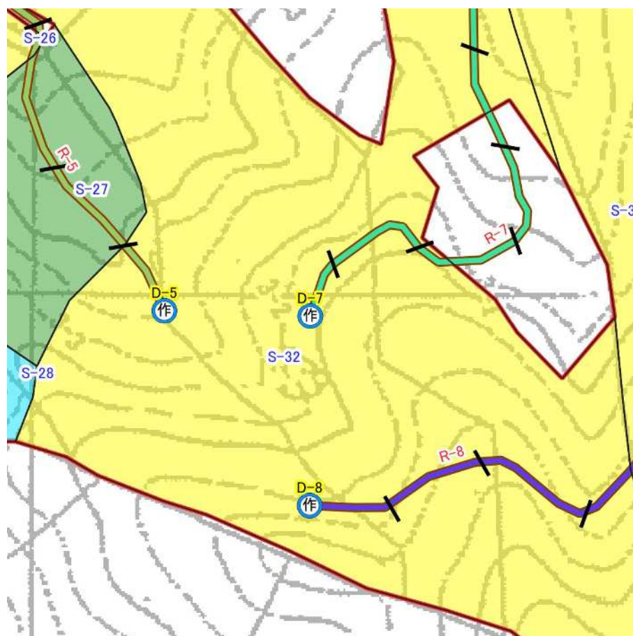
図表 5-10-1 D-7 標準平面図
