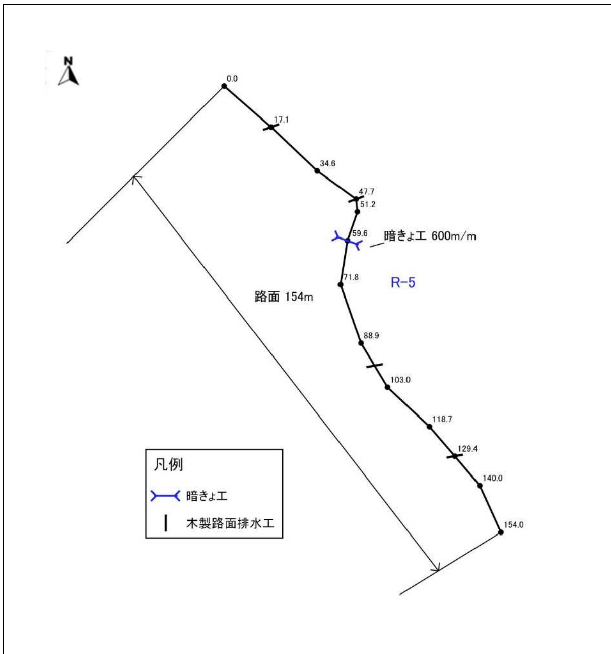
図表 4-5-1 R-5 の平面図(1)
