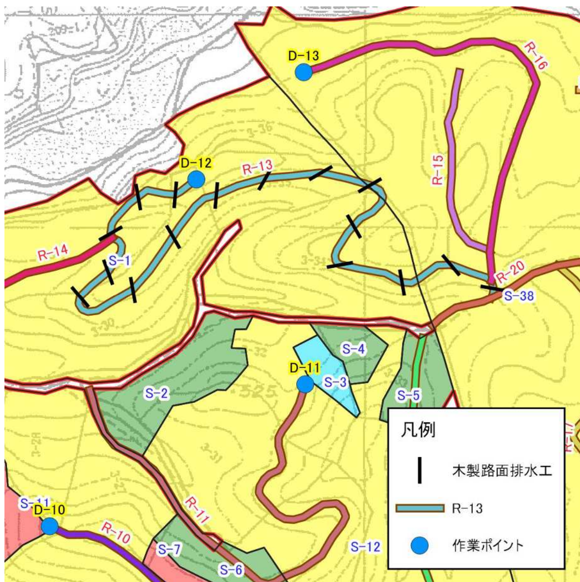
図表 4-13-3 R-13 の平面図(2)
