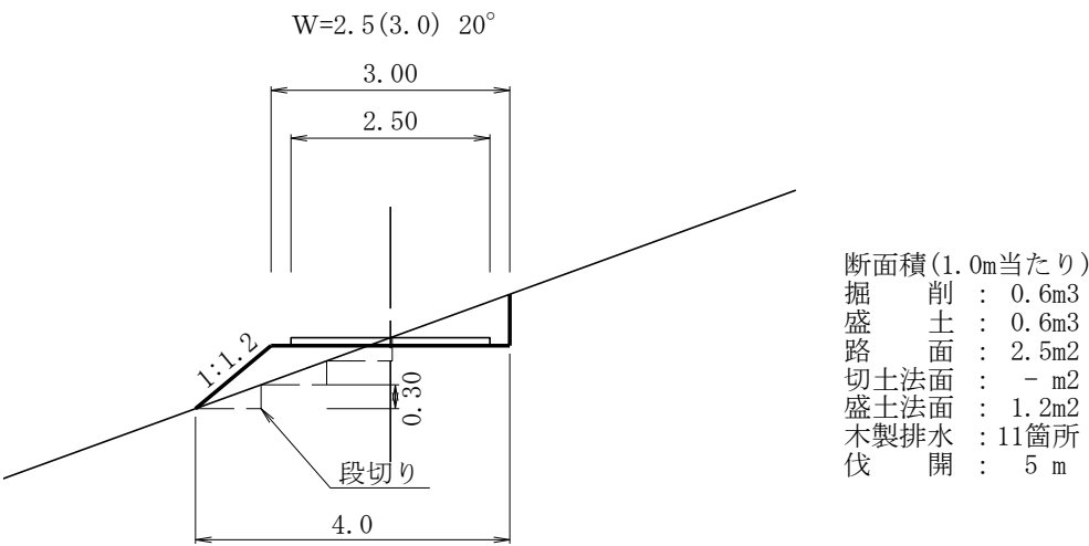
R-8標準横断図
