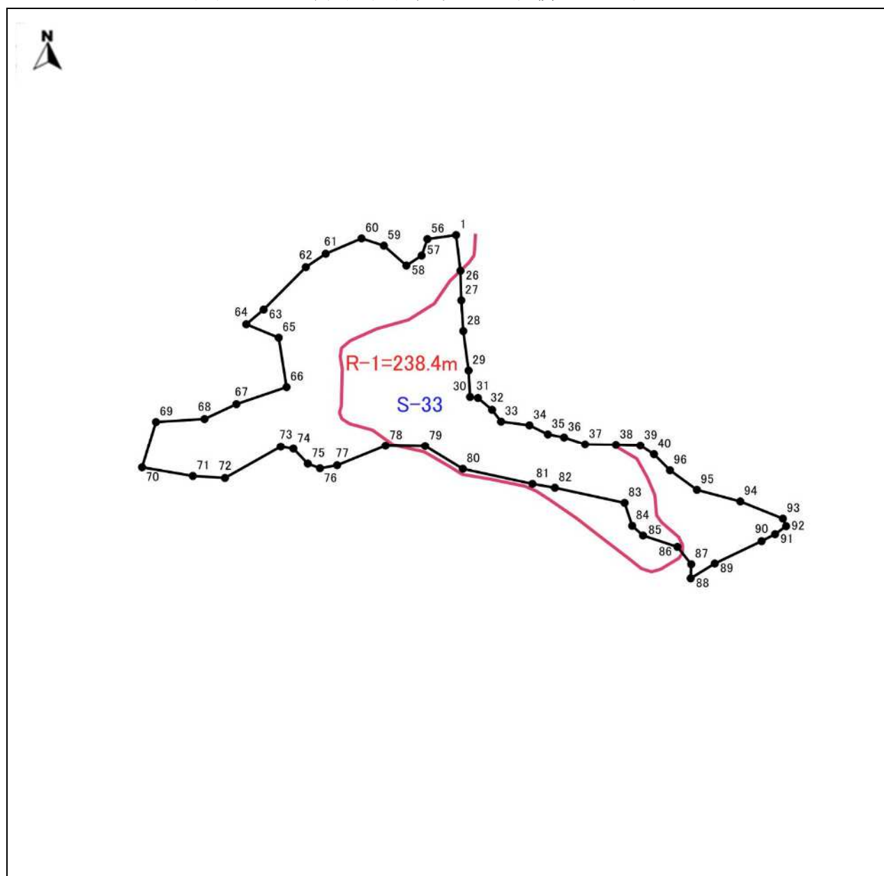
図表 1-36-1 平面図(地区番号：S-33 面積：2.10ha)
