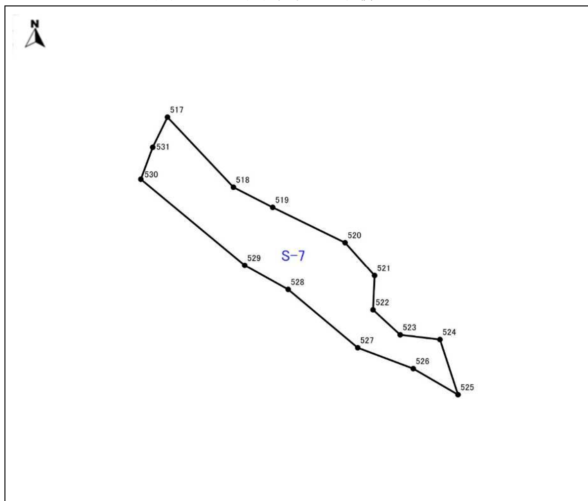
図表 1-10-1 (地区番号 : S-7 面積 : 0.16ha)
