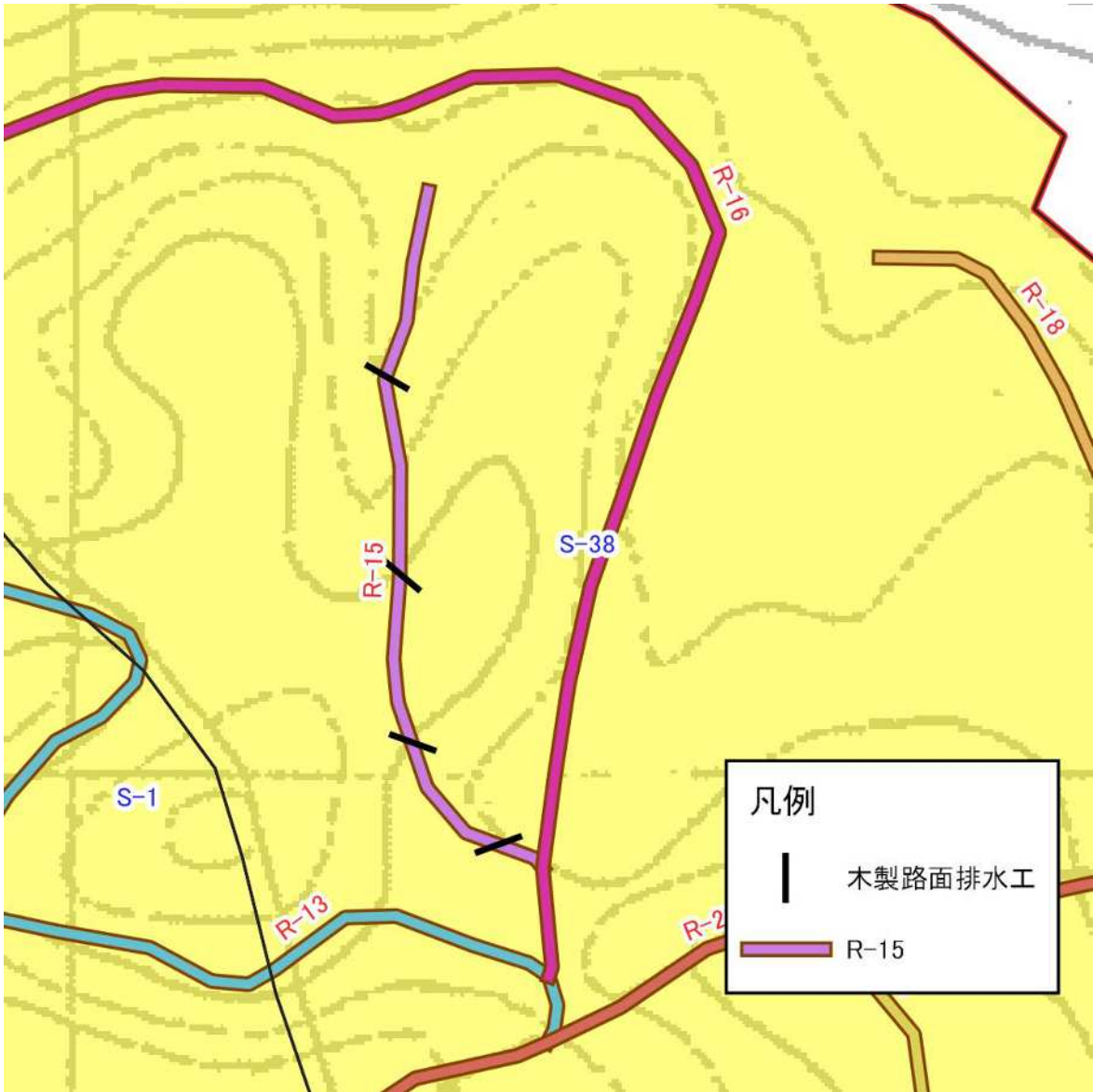
図表 4-15-3 R-15 の平面図(2)
