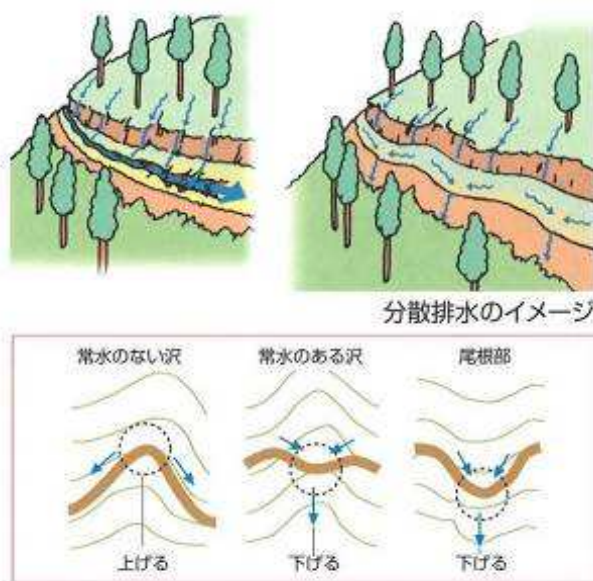
図表 5-1-6 波状勾配による分散排水
