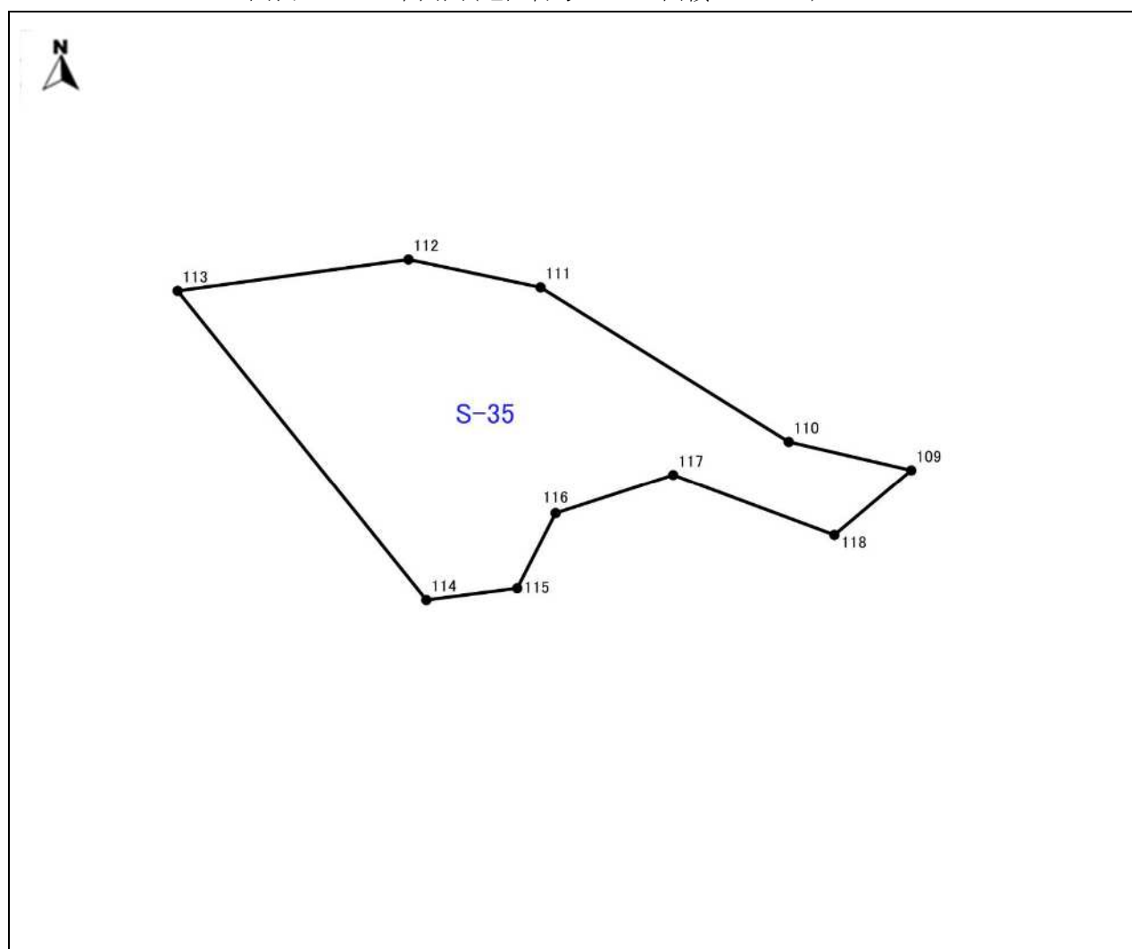
図表 1-38-1 平面図(地区番号 : S-35 面積 : 0.06ha)
