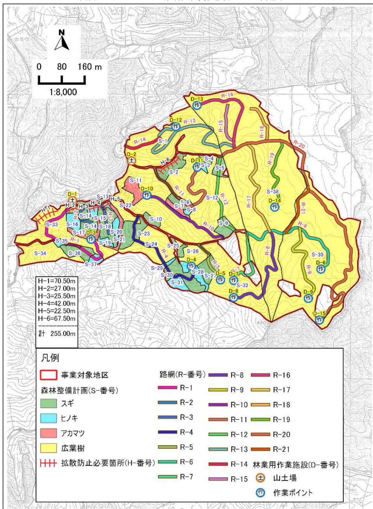
図表 3-1 H-1～H-6 の放射性物質拡散防止工の平面図
