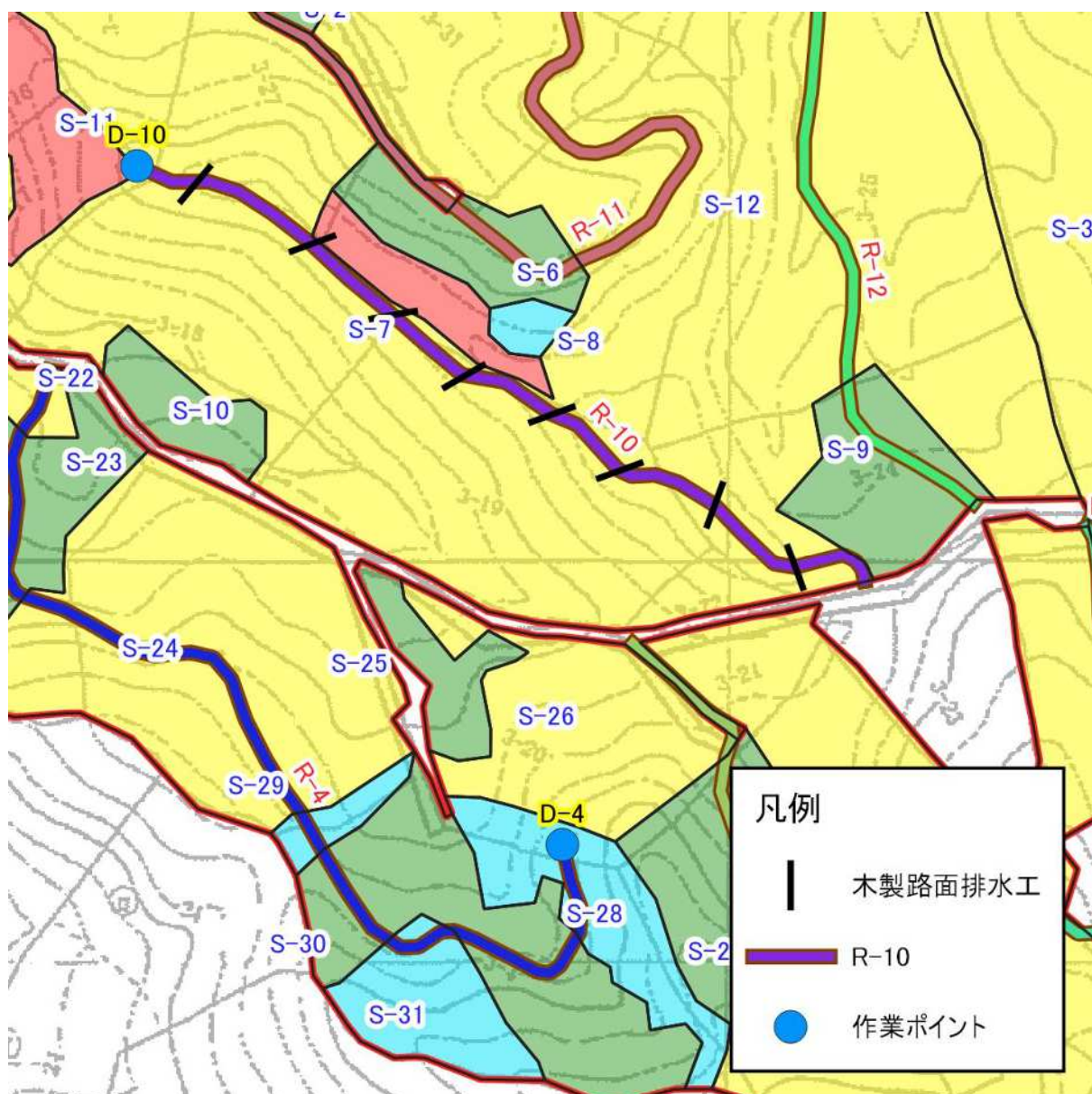
図表 4-10-3 R-10 の平面図(2)
