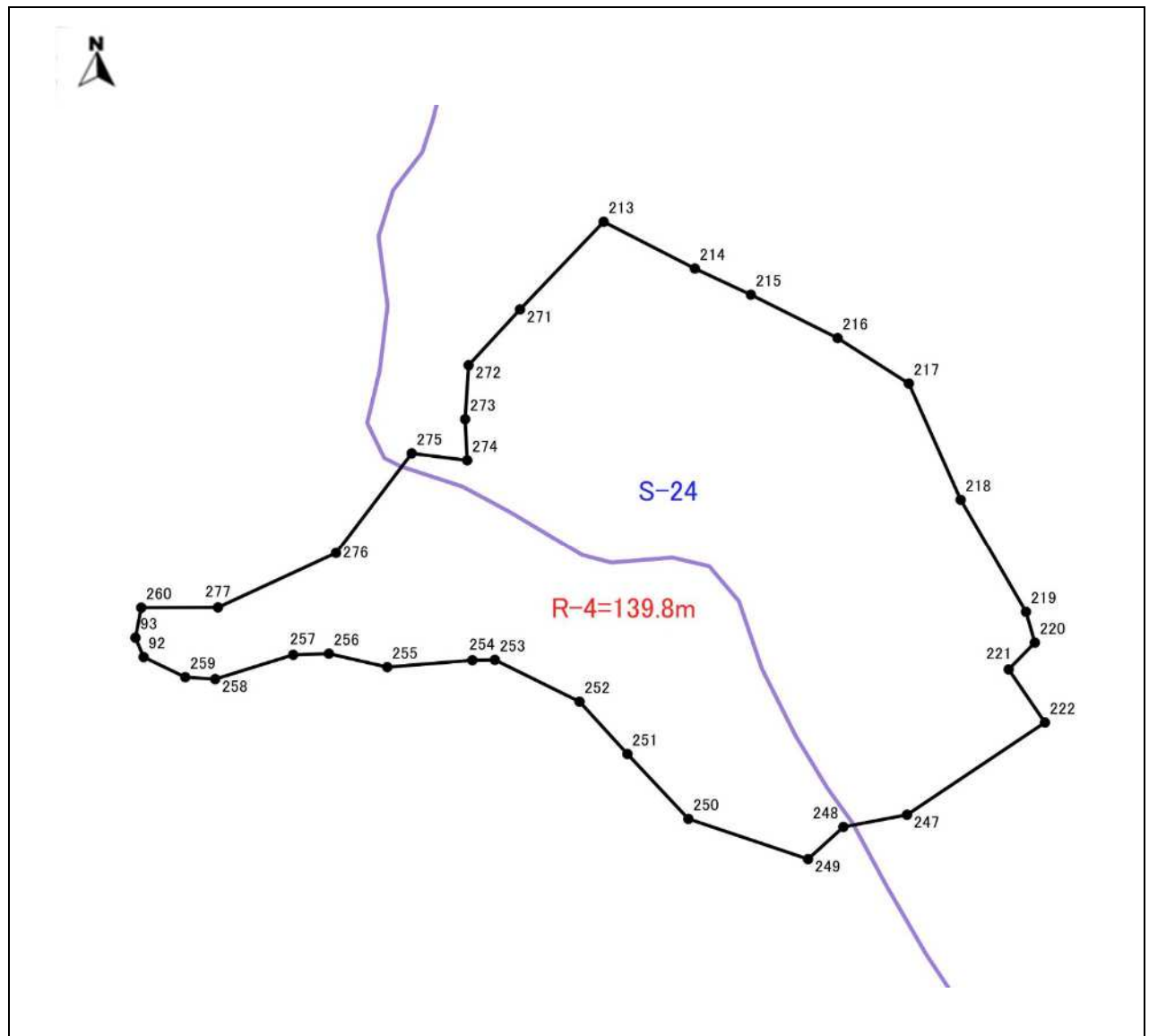
図表 1-27-1 平面図(地区番号：S-24 面積：1.38ha)
