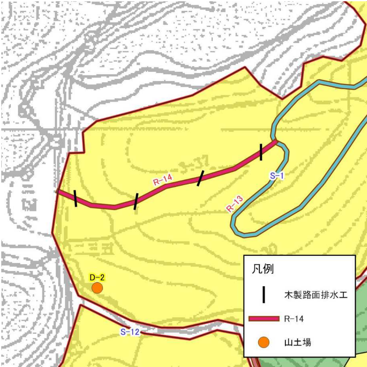
図表 4-14-3 R-14 の平面図(2)
