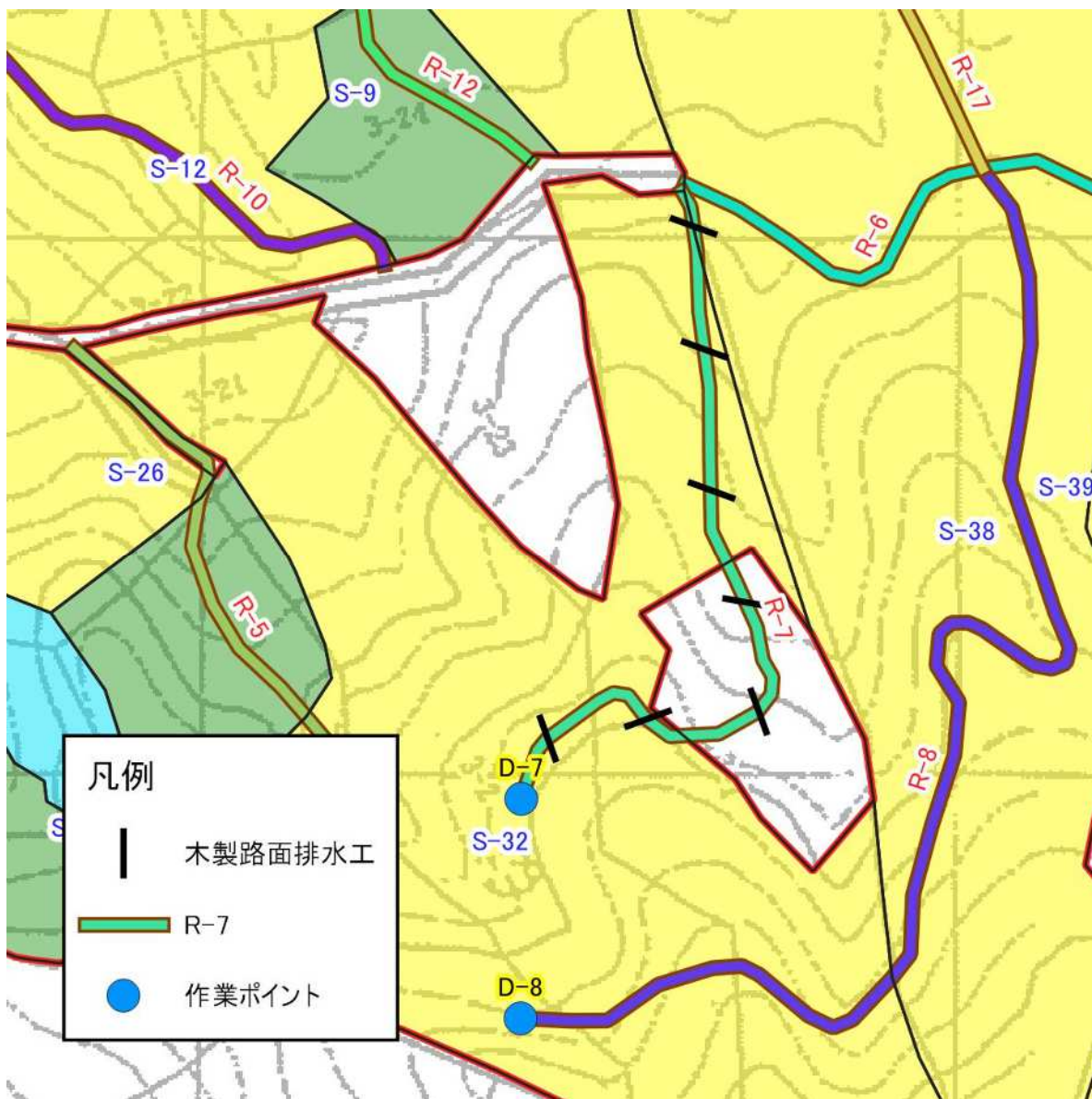
図表 4-7-3 R-7 の平面図(2)
