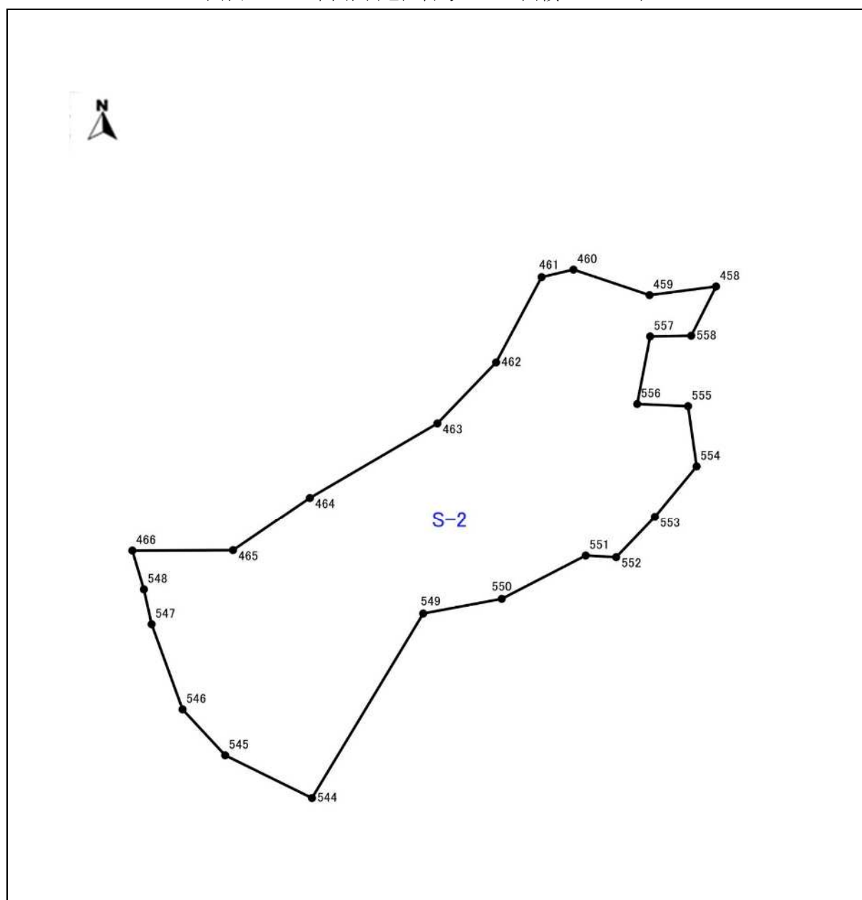
図表 1-5-1 平面図(地区番号 : S-2 面積 : 0.45ha)
