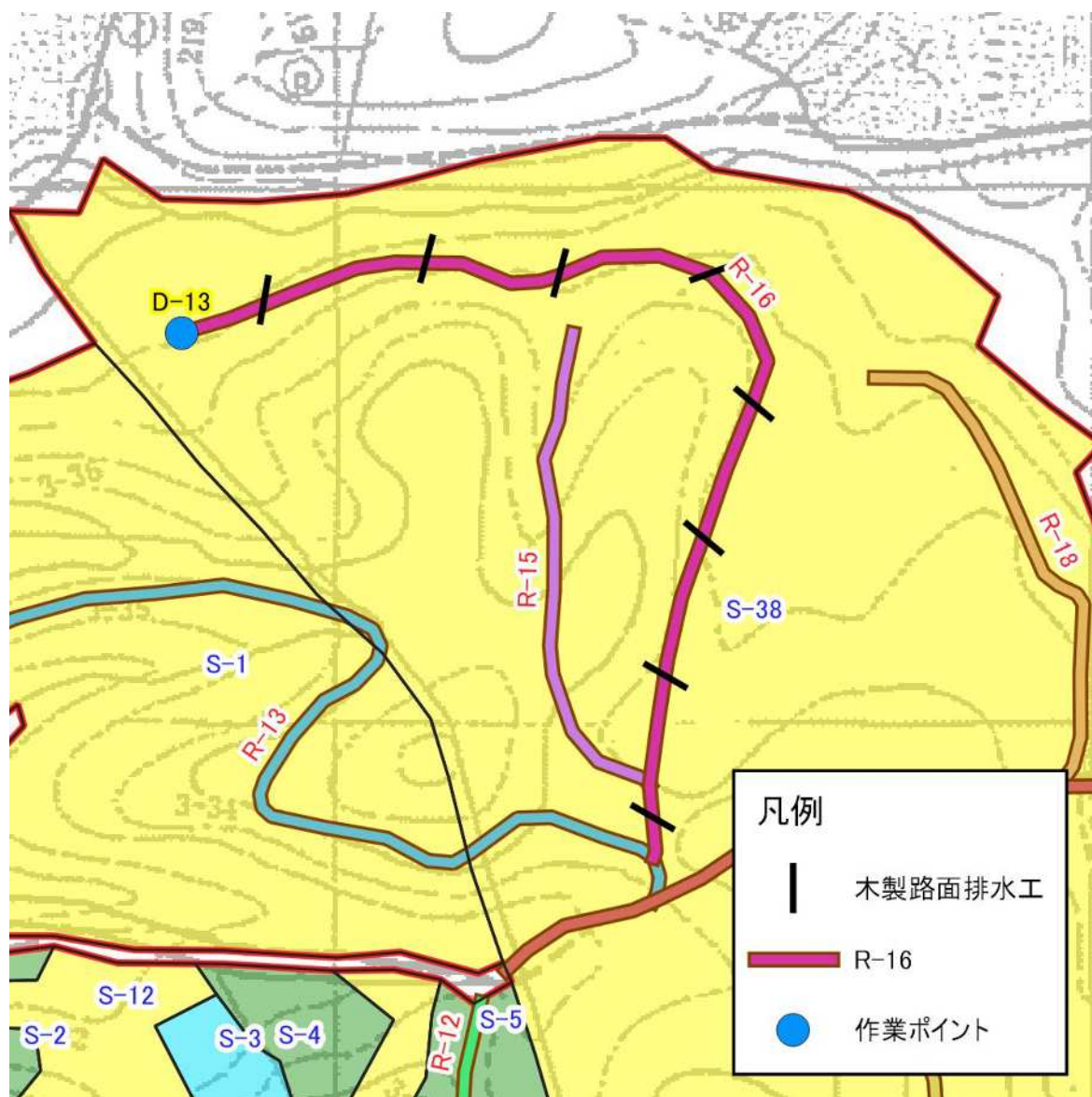
図表 4-16-3 R-16 の平面図(2)
