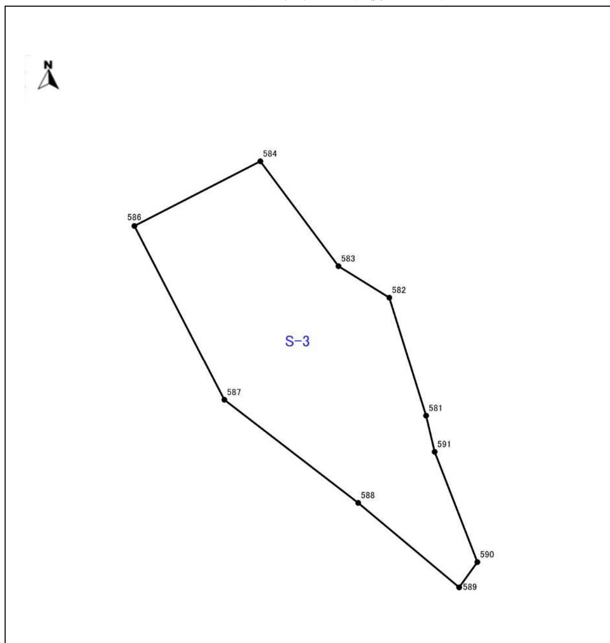
図表 1-6-1 (地区番号 : S-3 面積 : 0.11ha)
