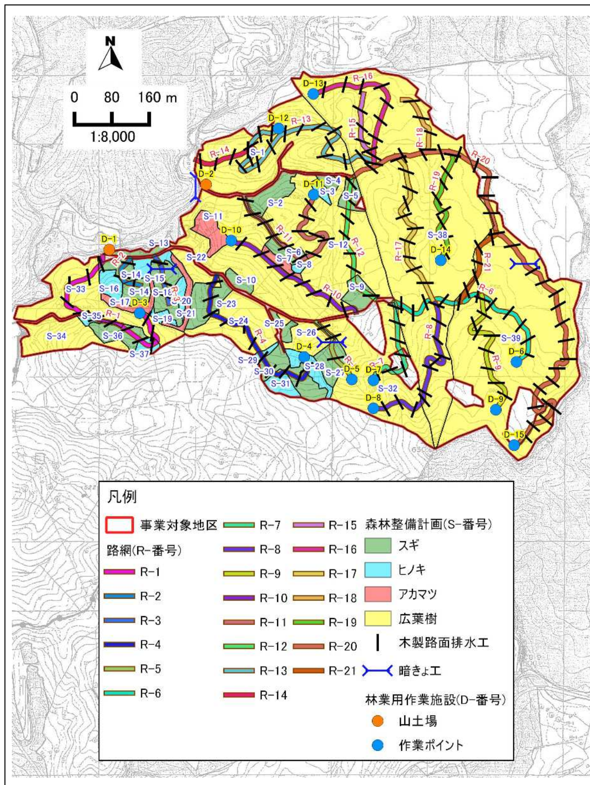
図表 5-3-1 D-1～D-15 平面図
