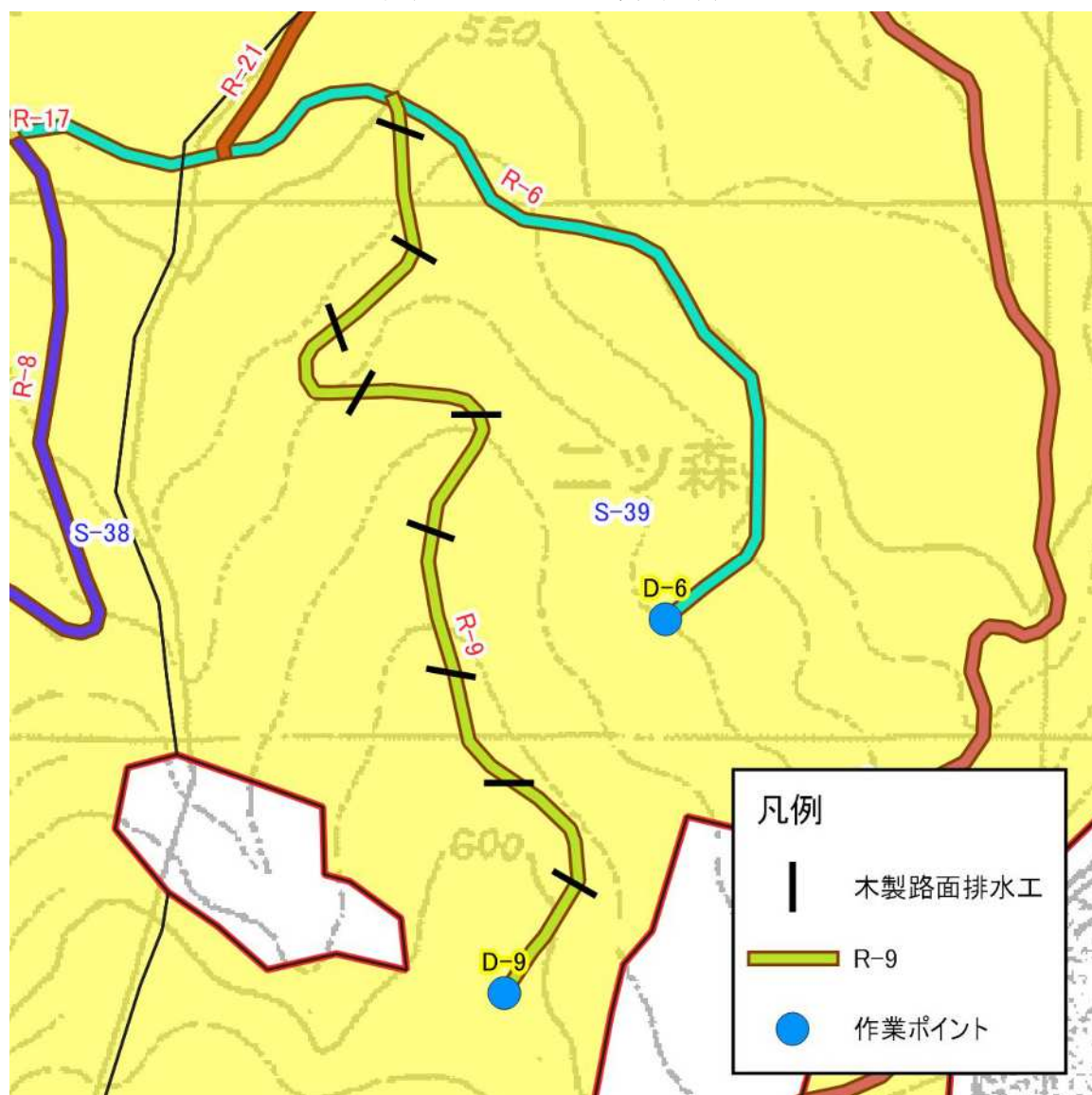
図表 4-9-3 R-9 の平面図(2)
