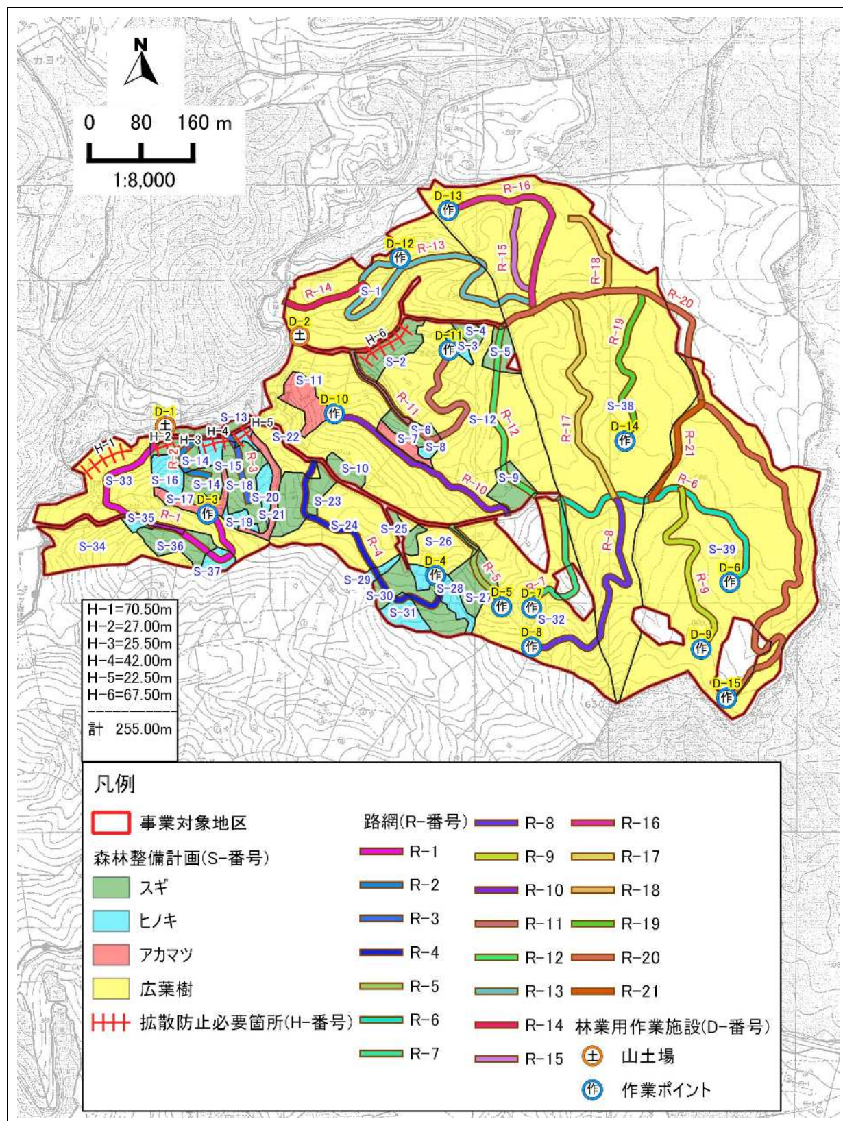
図表 3-3-1 放射性物質拡散防止の計画図
