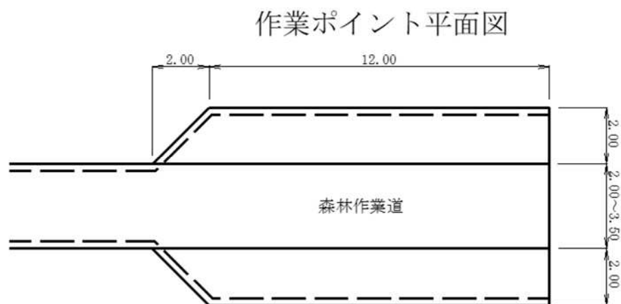
図表 5-8-2 D-5 標準平面図
