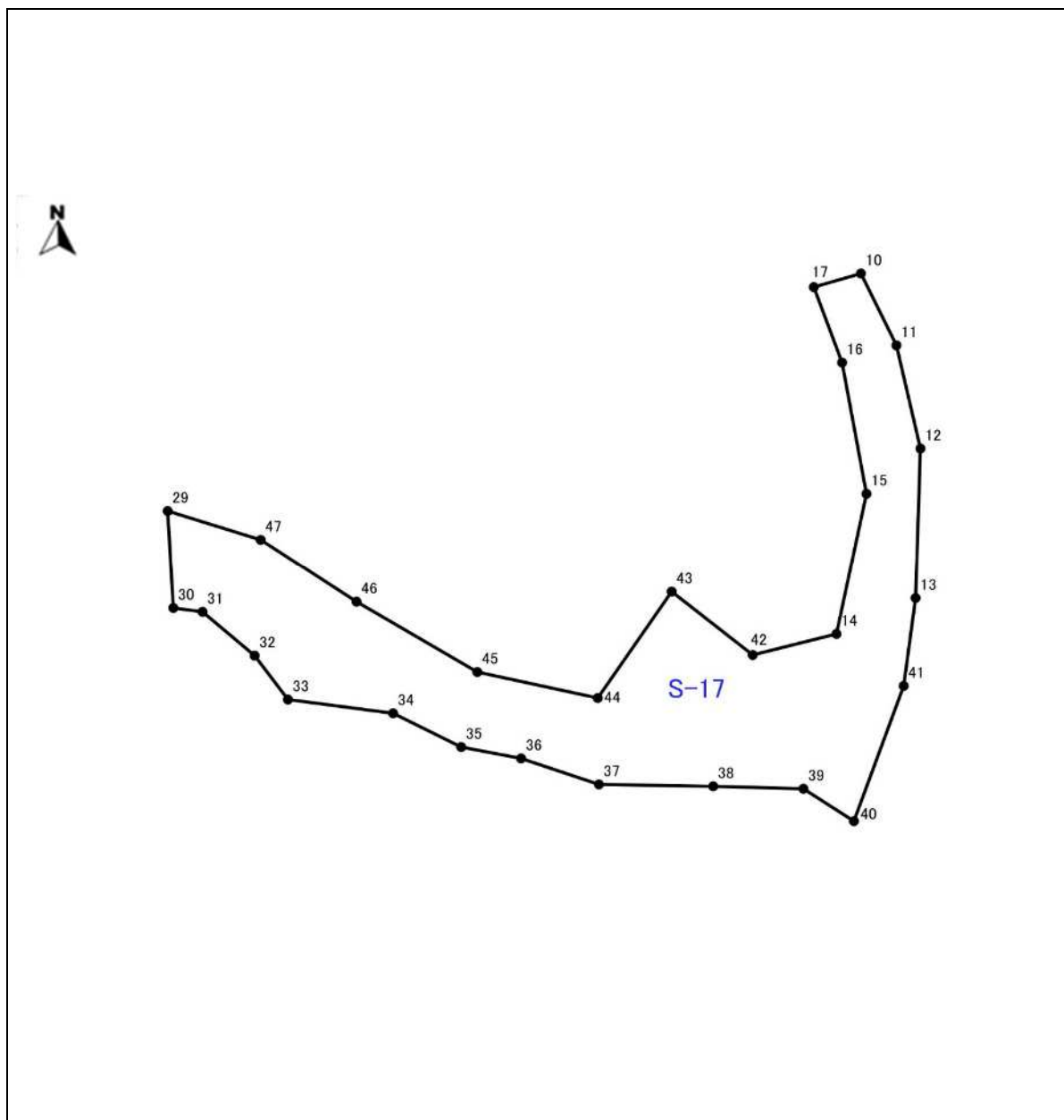
図表 1-20-1 (地区番号 : S-17 面積 : 0.26ha)
