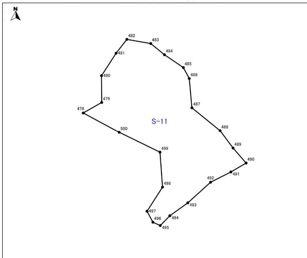
図表 1-14-1 平面図(地区番号 : S-11 面積 : 0.38ha)
