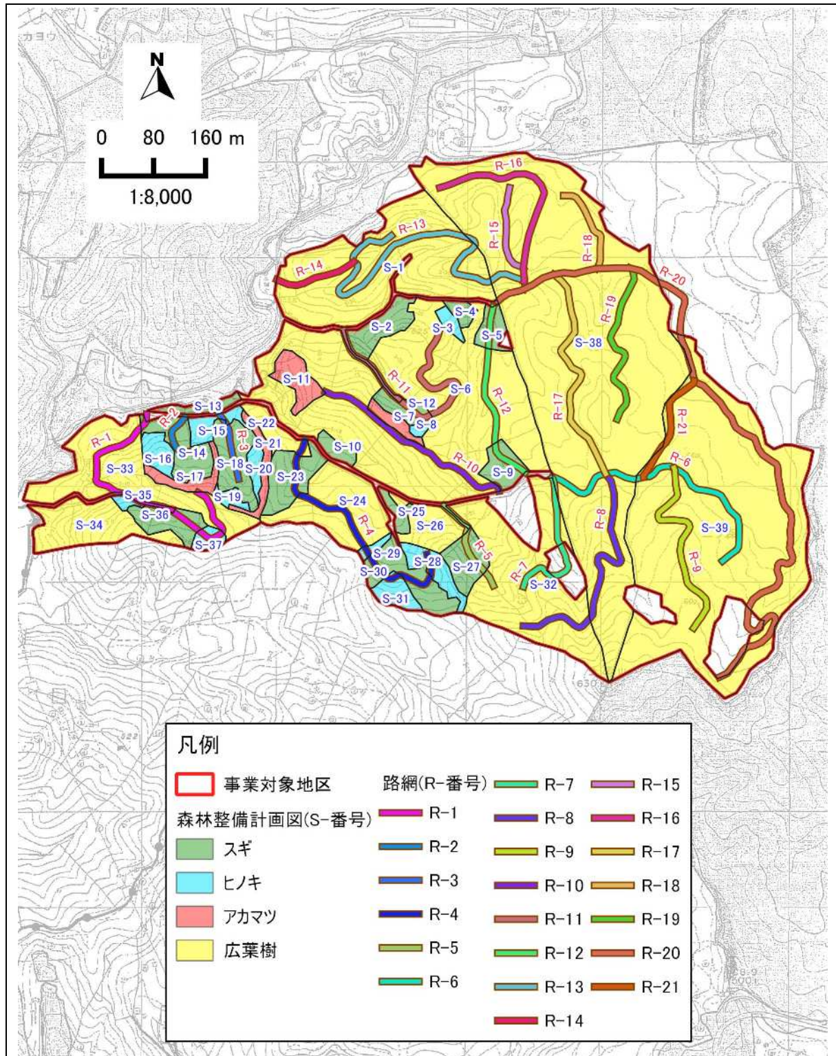
図表 4-1 路網整備の平面図
