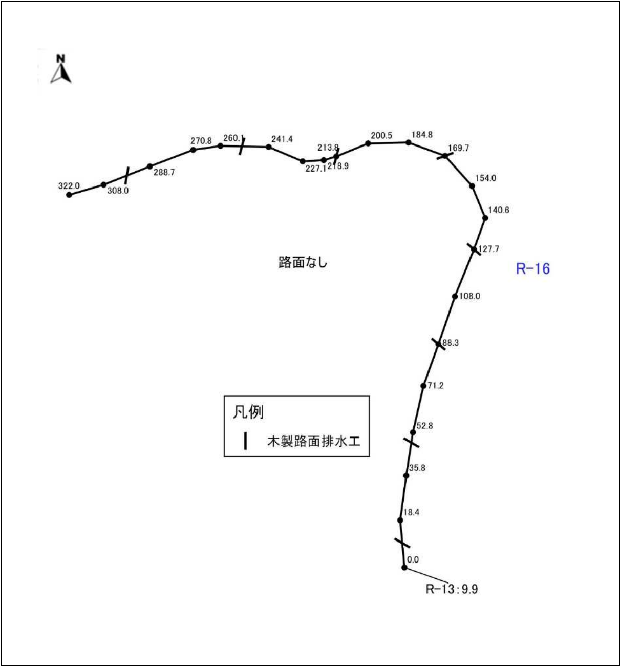
図表 4-16-1 R-16 の平面図 (1)
