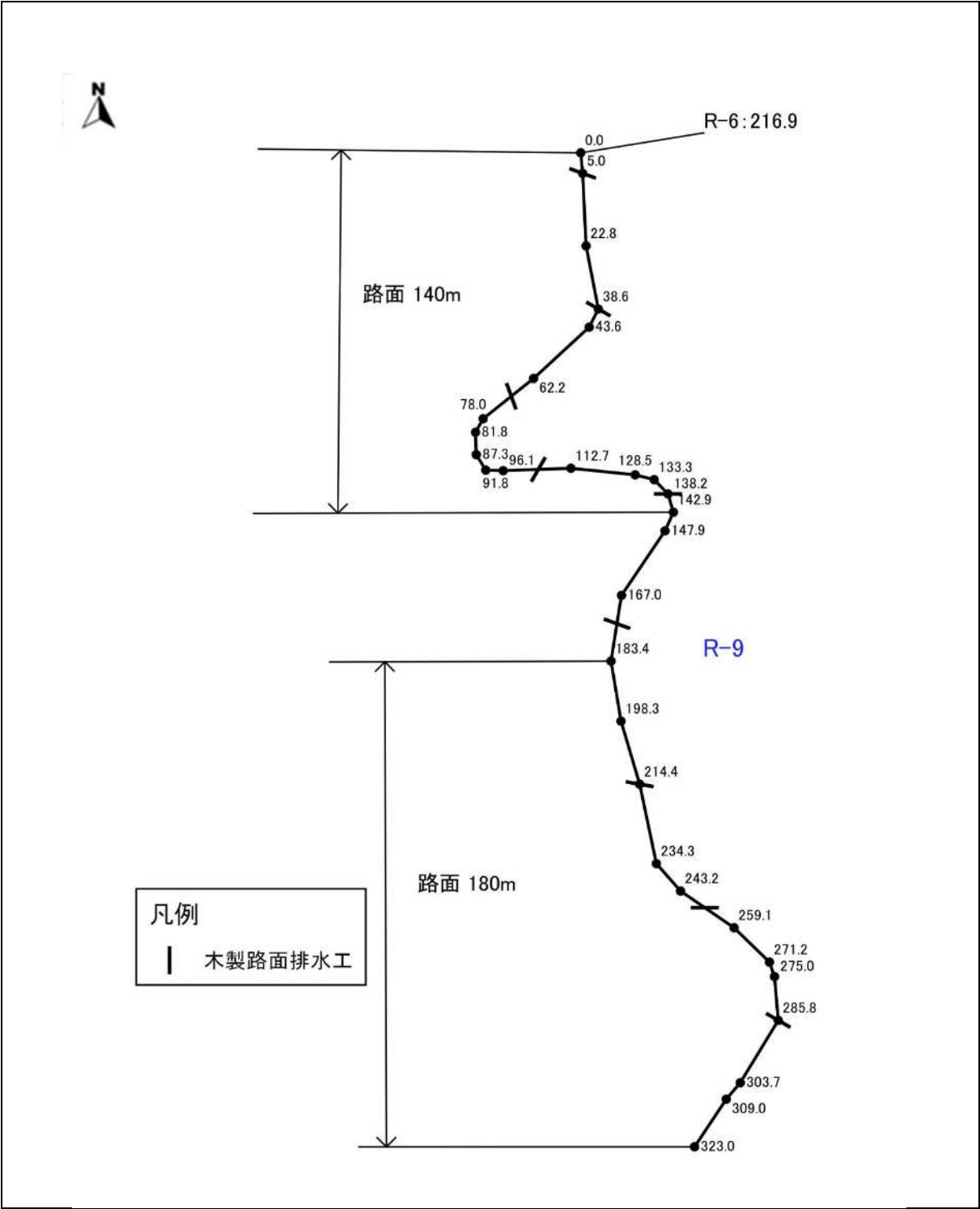
図表 4-9-1 R-9 の平面図(1)
