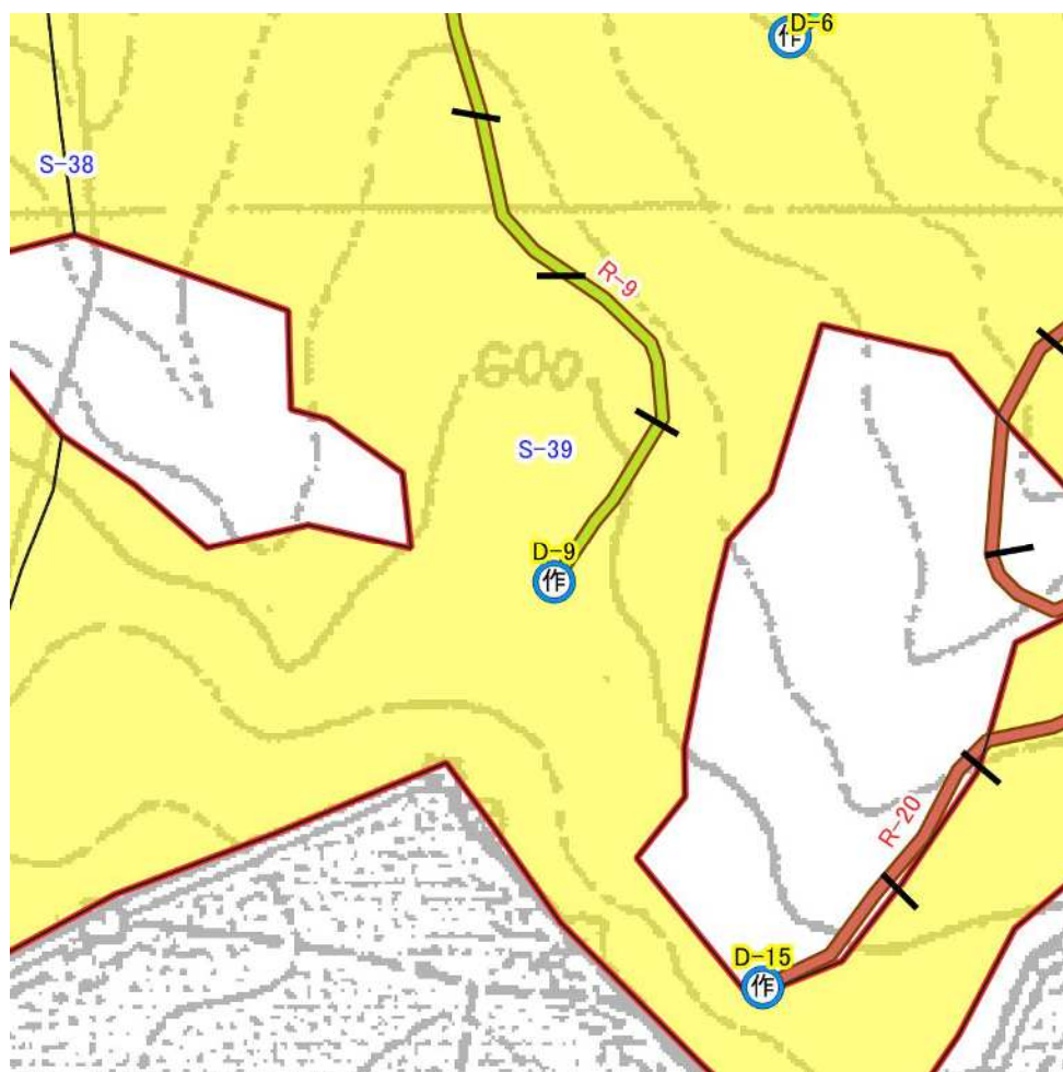
図表 5-12-1 D-9 平面図
