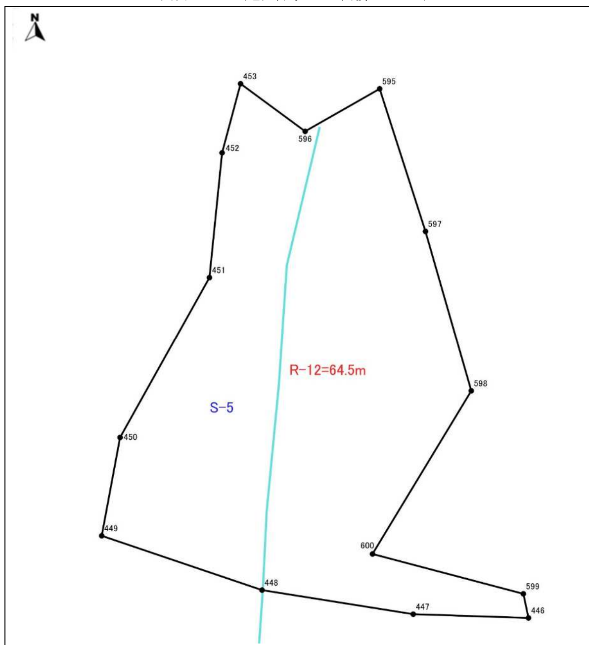
図表 1-8-1 (地区番号 : S-5 面積 : 0.25ha)
