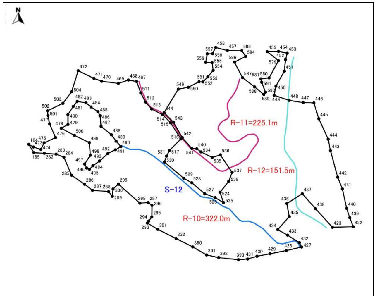
図表 1-15-1 平面図(地区番号 : S-12 面積 : 7.60ha)
