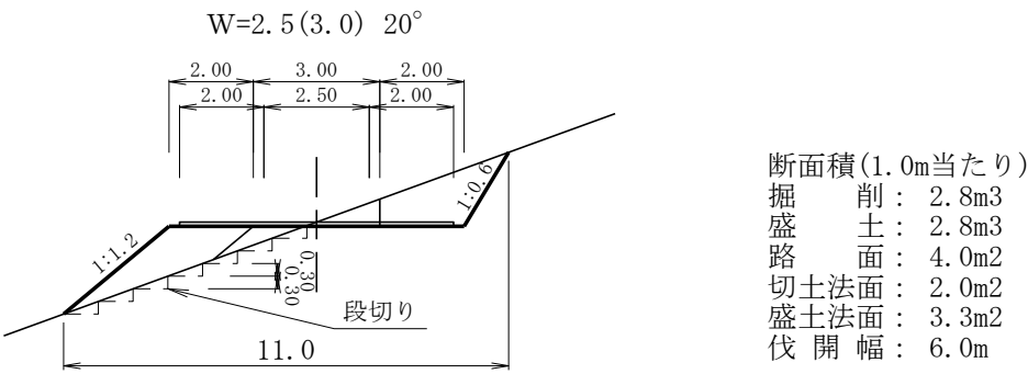
作業ポイント横断図(D-4)
