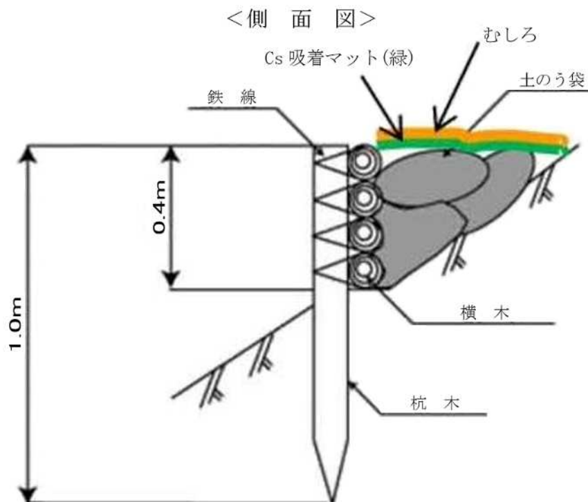
図表 3-2-5 吸着材使用の標準図
