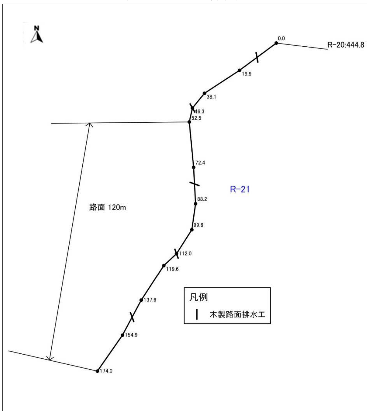
図表 4-21-1 R-21 の平面図(1)
