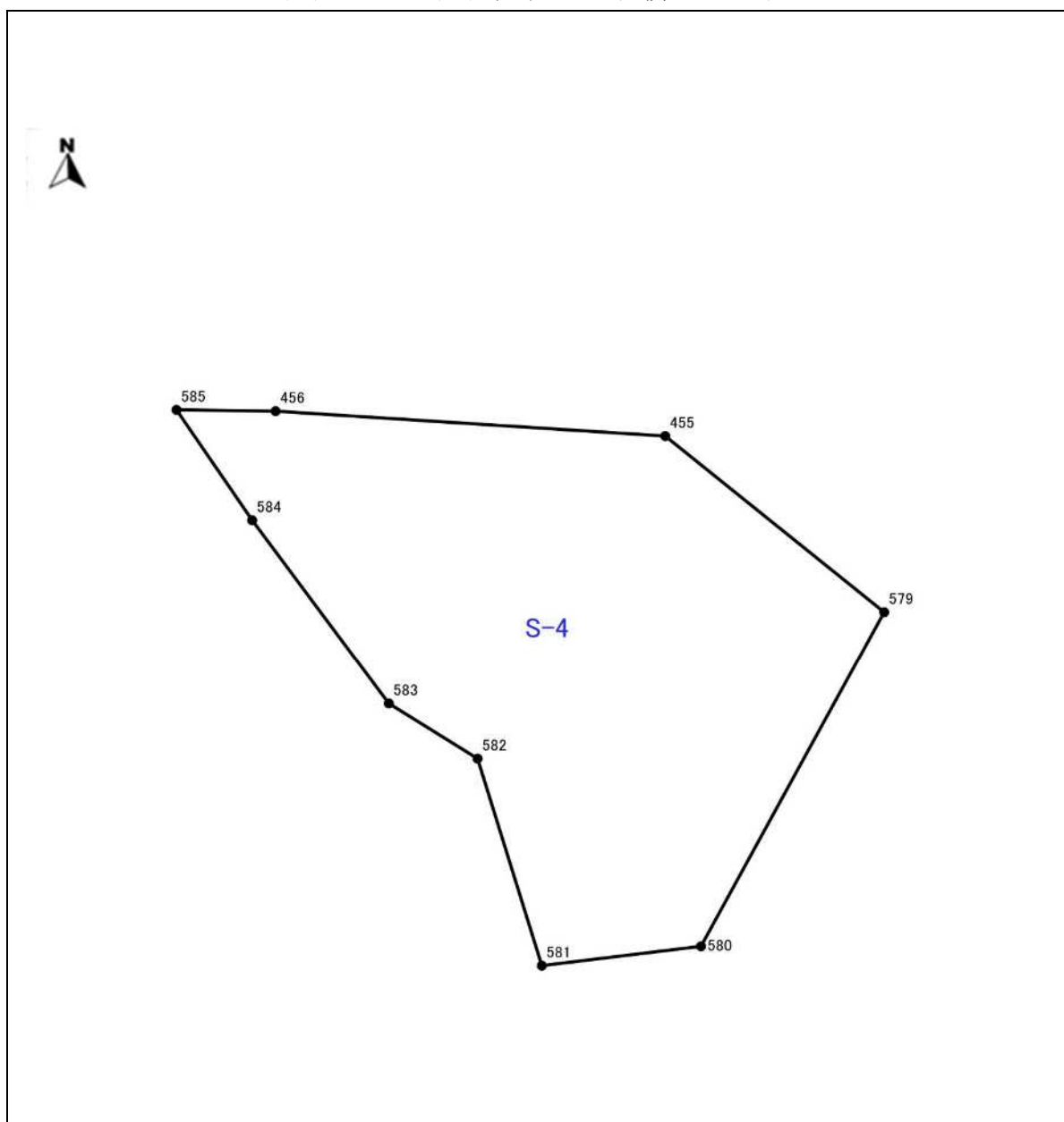
図表 1-7-1 (地区番号 : S-4 面積 : 0.13ha)
