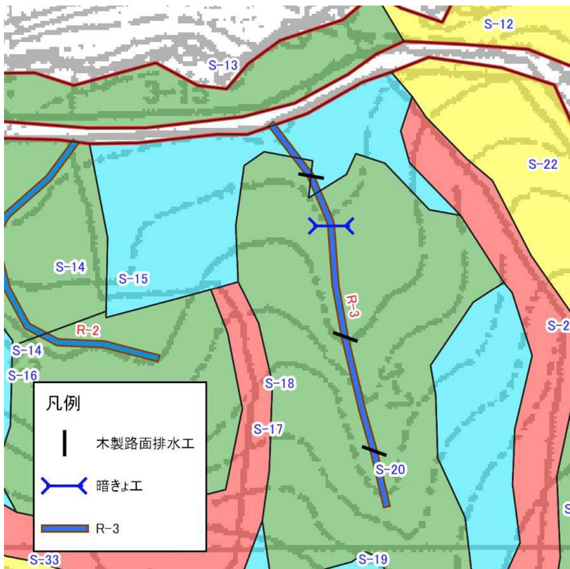
図表 4-3-3 R-3 の平面図(2)
