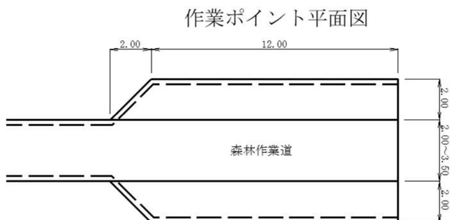
図表 5-14-2 D-11 標準平面図
