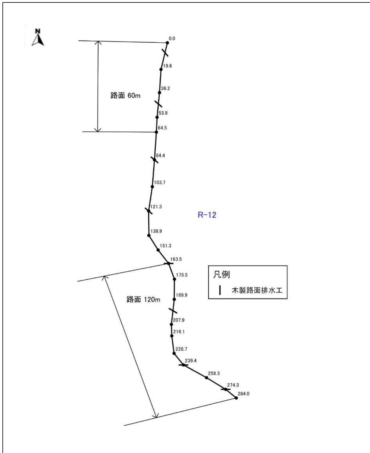
図表 4-12-1 R-12 の平面図(1)
