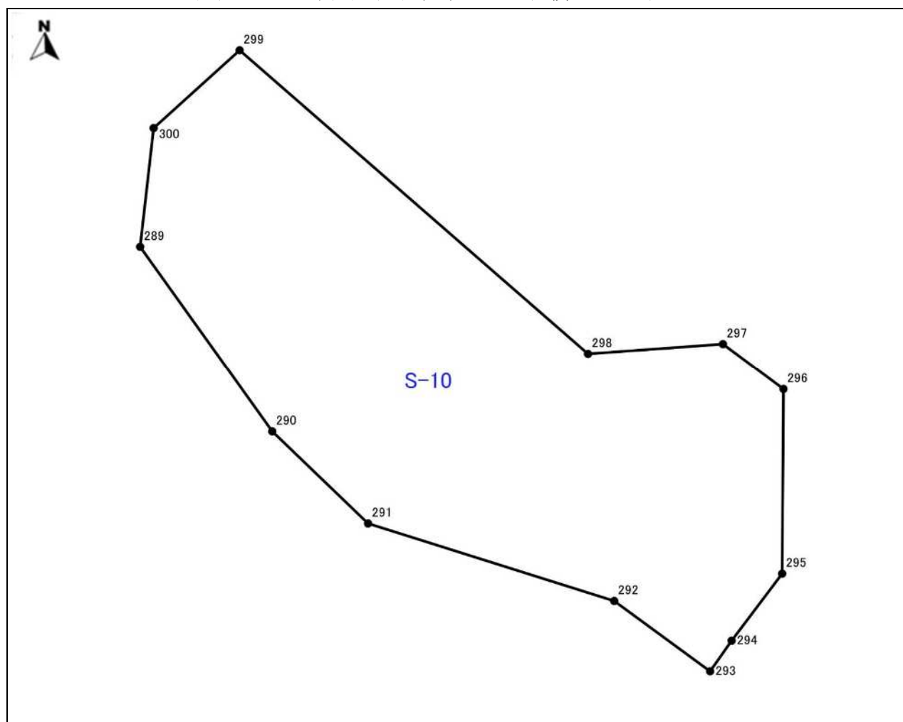
図表 1-13-1 平面図(地区番号 : S-10 面積 : 0.16ha)
