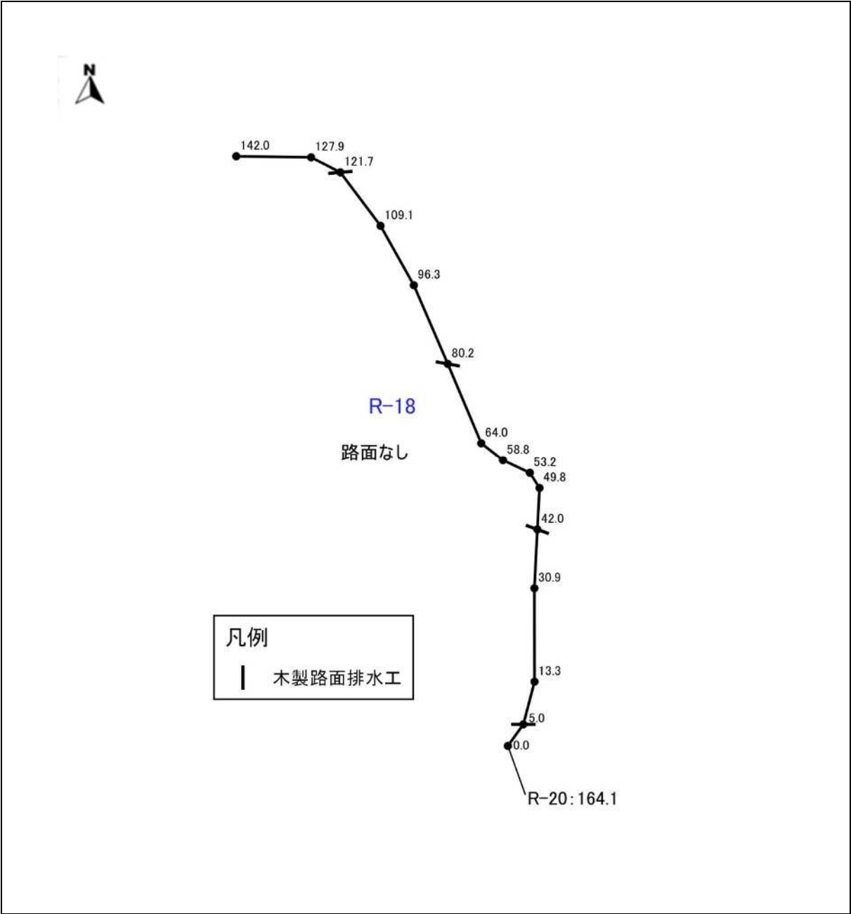
図表 4-18-1 R-18 の平面図 (1)
