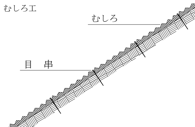
図表 3-2-3 伏工標準図
