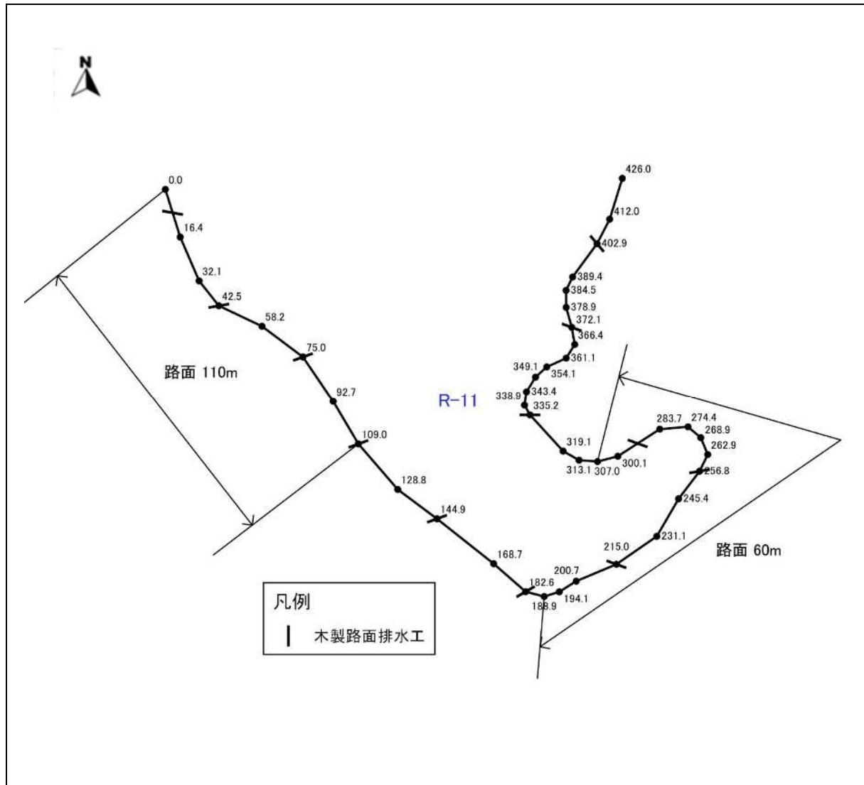
図表 4-11-1 R-11 の平面図(1)
