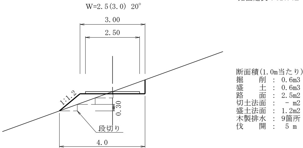
R-9標準横断図
