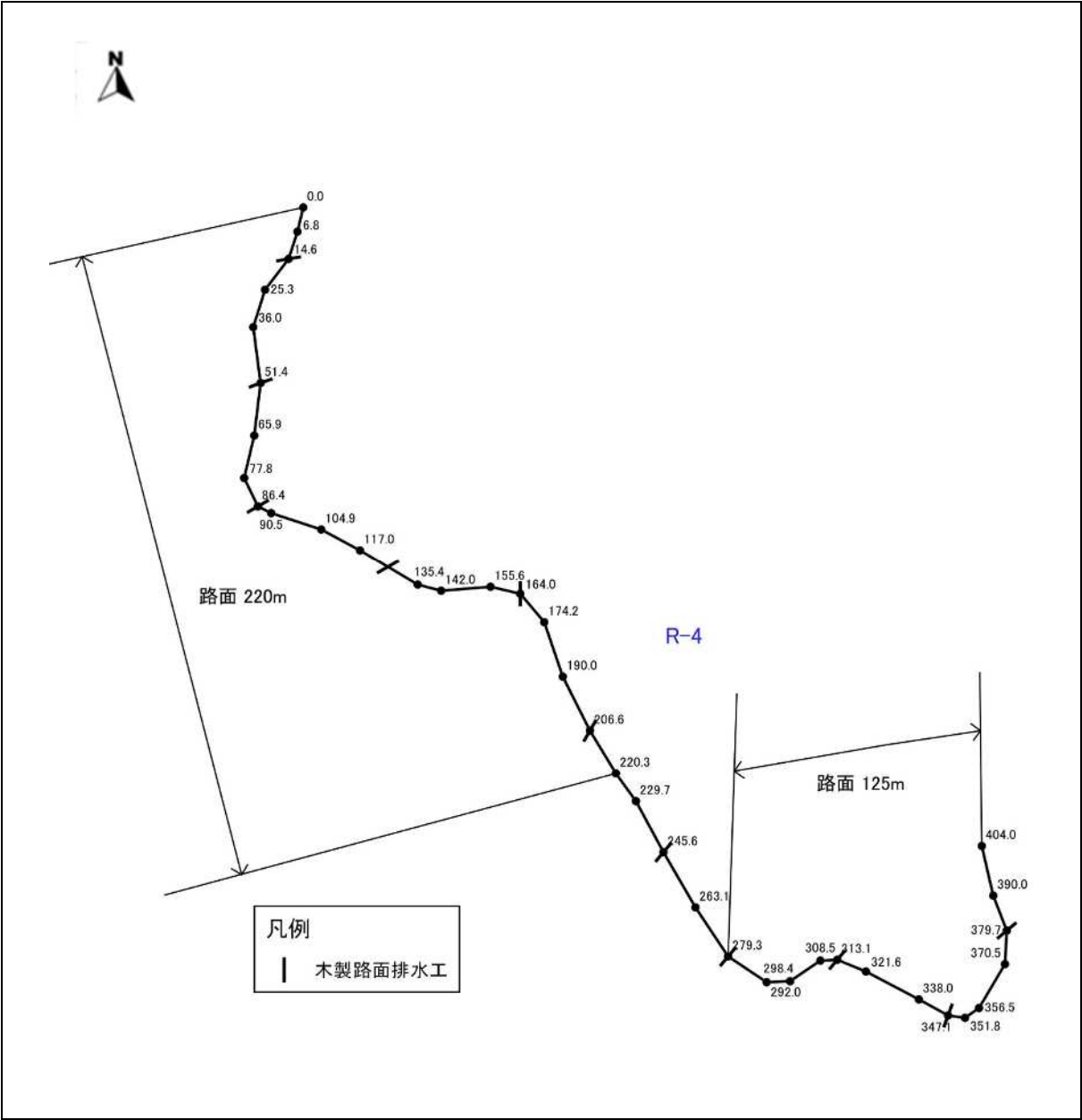
図表 4-4-1 R-4 の平面図(1)
