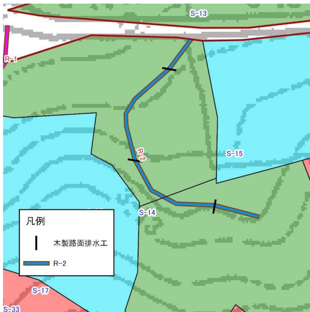
図表 4-2-3 R-2 の平面図(2)
