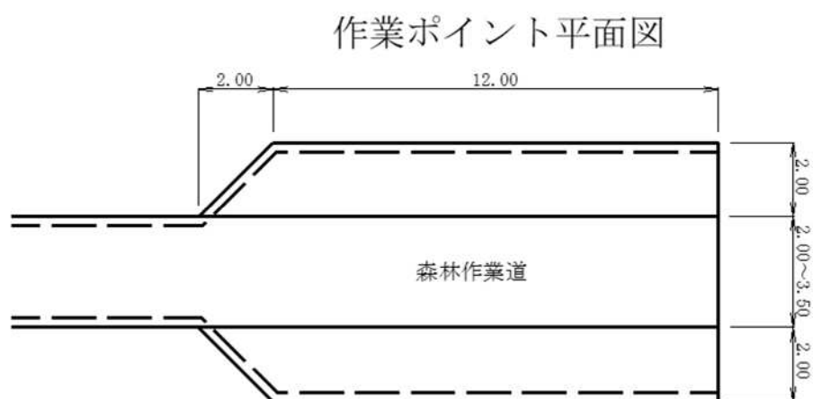
図表 5-11-2 D-8 標準平面図
