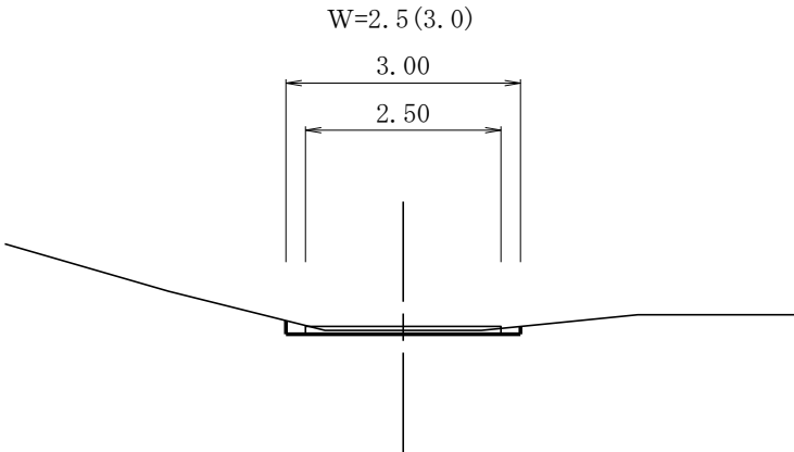
R-6標準横断面図
