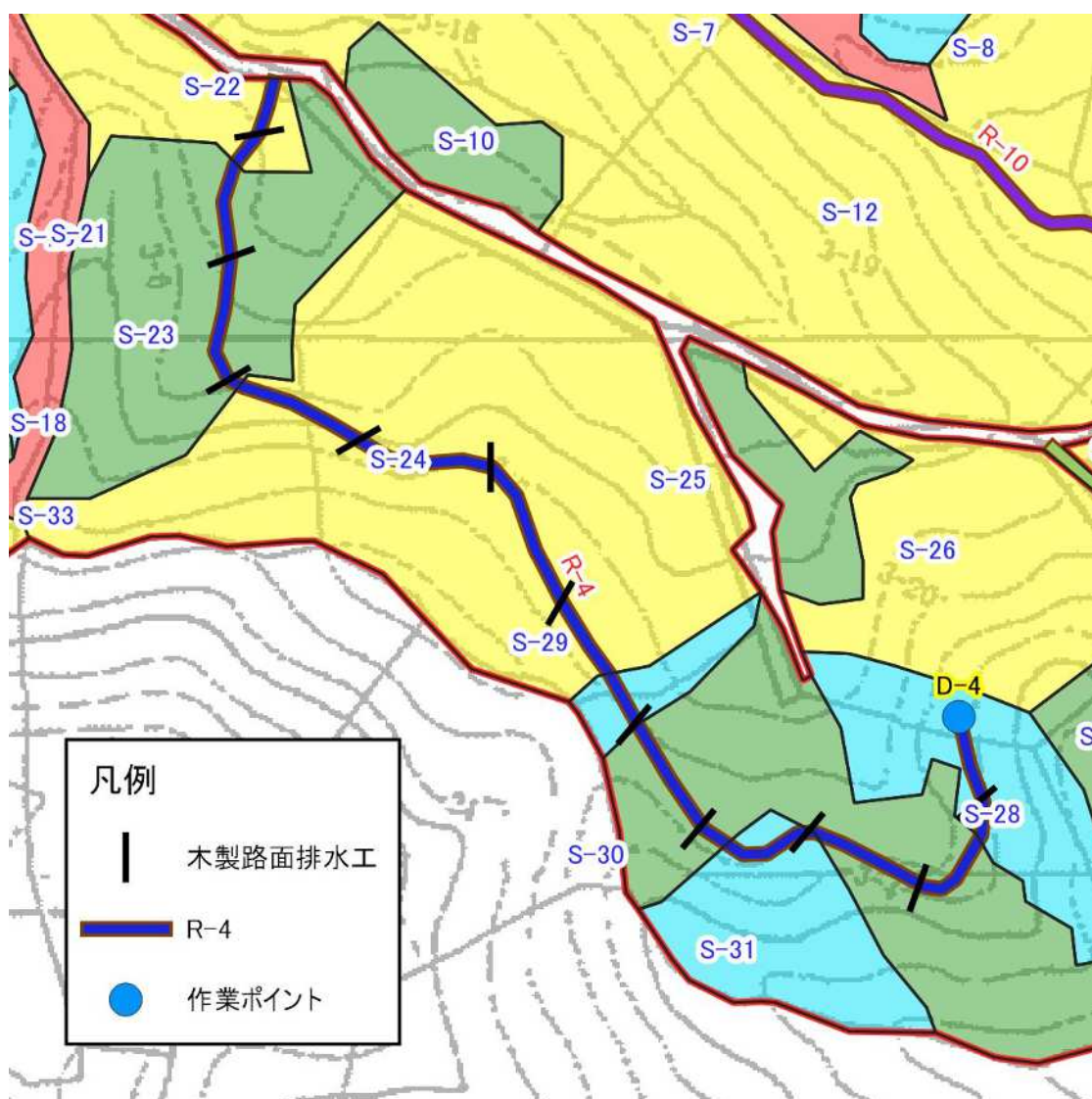
図表 4-4-3 R-4 の平面図(2)
