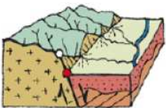
ずれ断層
