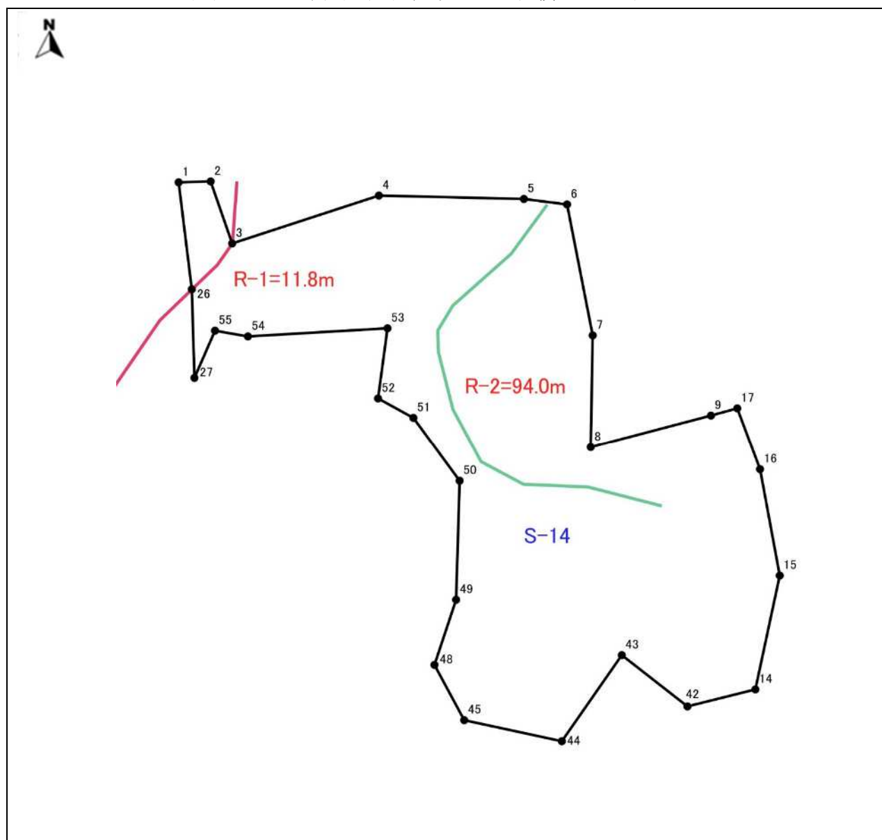
図表 1-17-1 平面図(地区番号 : S-14 面積 : 0.57ha)
