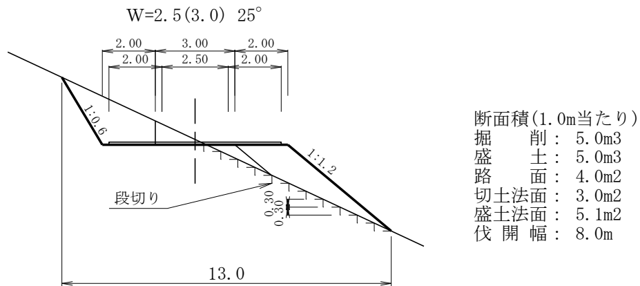
作業ポイント横断図(D-7)
