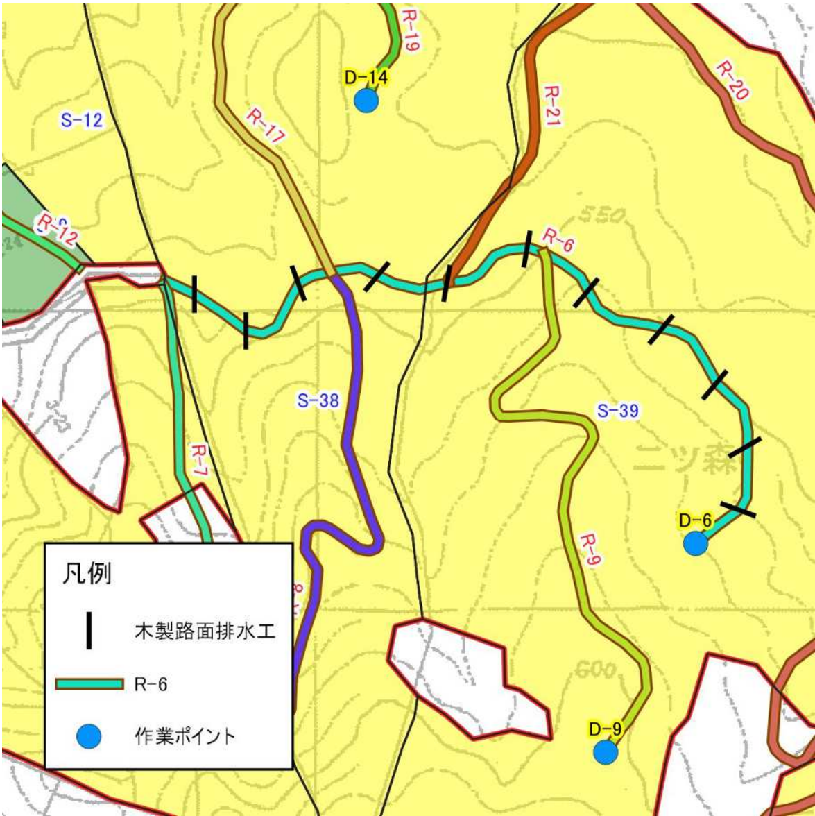
図表 4-6-3 R-6 の平面図(2)
